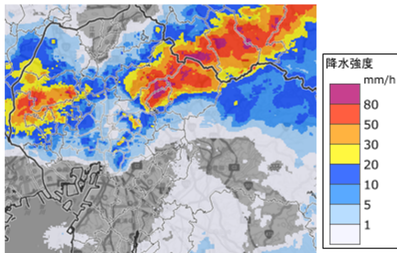
高解像度降水ナウキャスト 13日22時30分
