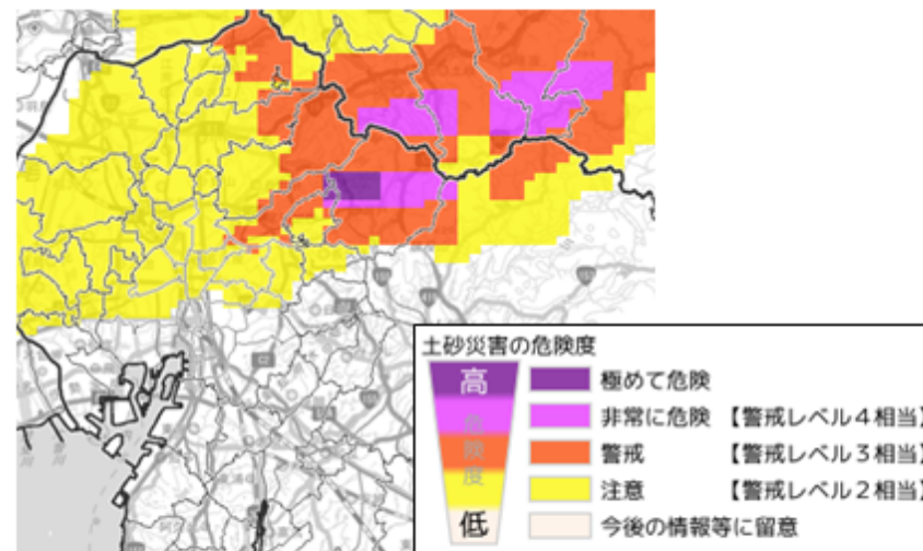
土砂キキクル(危険度分布) 13日22時30分
