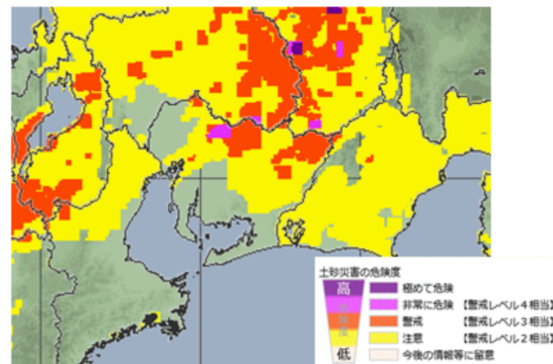
大雨警報(土砂災害)のキキクル(危険度分布) 21日8時20分
