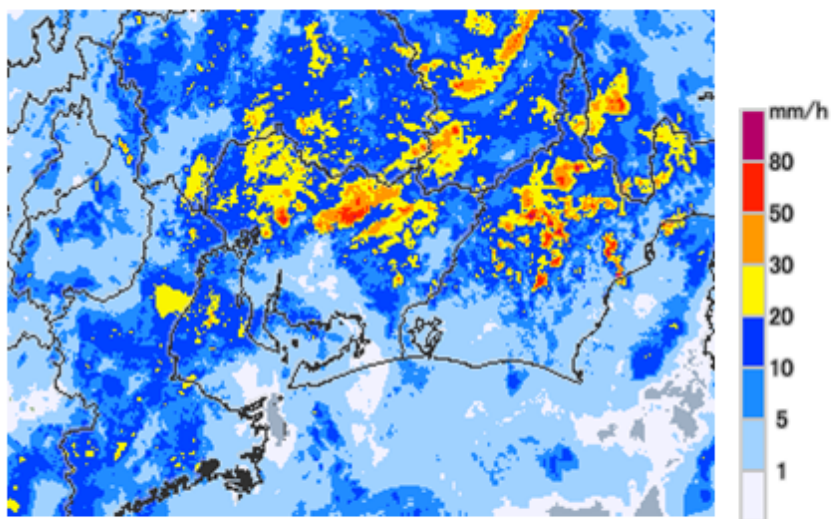
高解像度降水ナウキャスト 21日8時20分
