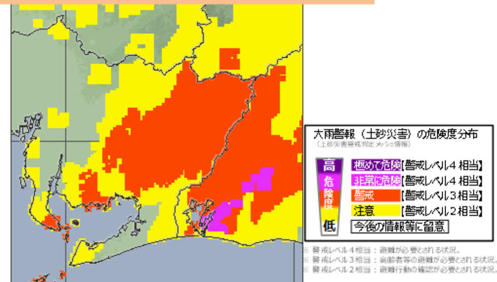
大雨警報(土砂災害)の危険度分布 26日17時30分
