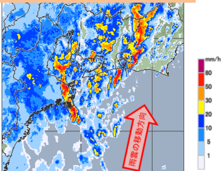
高解像度降水ナウキャスト 26日17時30分
