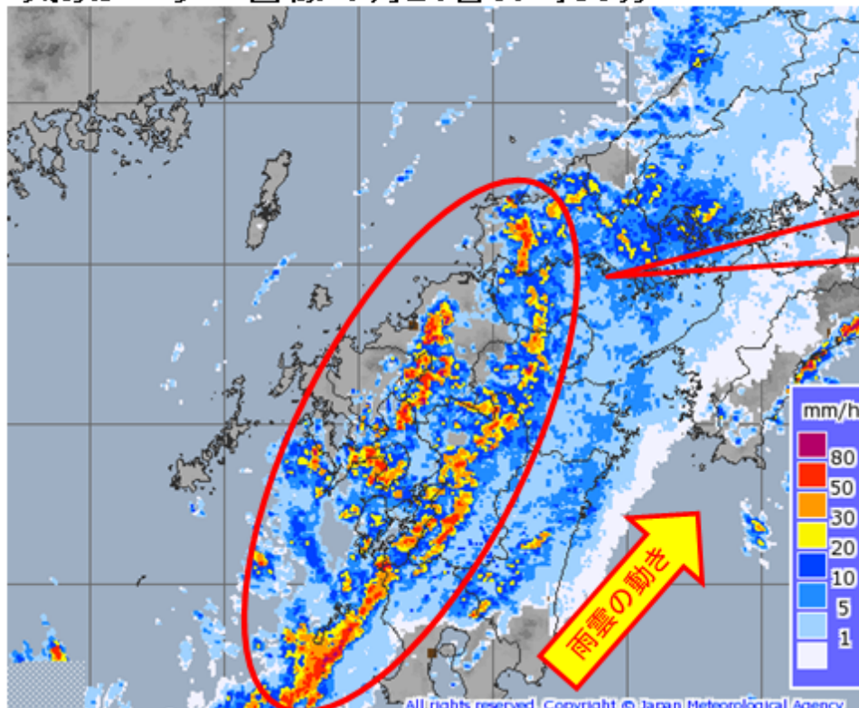
気象レーダー画像 7月24日07時30分
