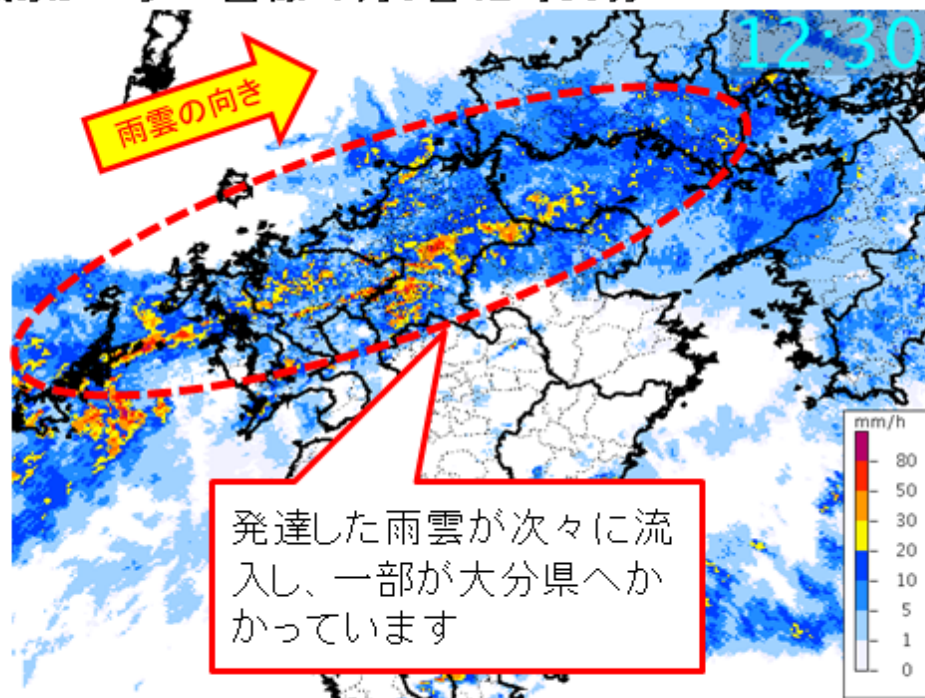
気象レーダー画像 7月6日12時30分
