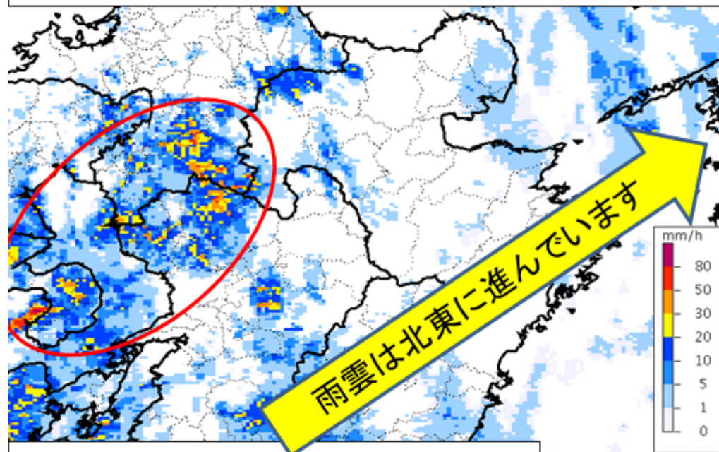
30日03時20分のレーダー実況図
