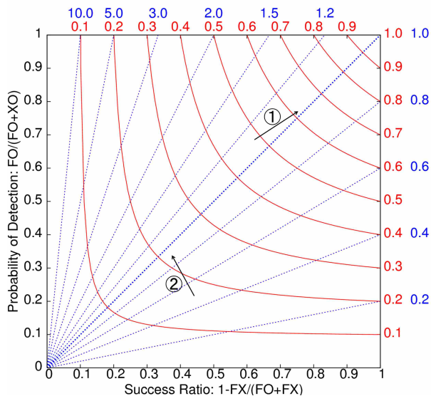
図 D.3.1 Roebber ダイアグラムの模式図。横軸は 1-空振り率、縦軸は捕捉率、青の破線はバイアスコアの、赤の実線はスレットスコアの各等値線。
