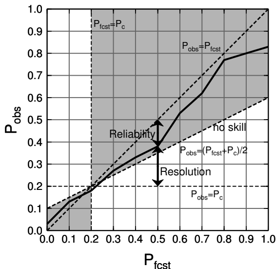
図 D.4.1 確率値別出現率図の模式図。横軸は予測現象出現確率、縦軸は実況現象出現相対頻度、実線が信頼度曲線である。対角線、直線 P_{obs} = P_c との差の二乗がそれぞれ信頼度 (Reliability)、分離度 (Resolution) への寄与に対応している。灰色の領域内の点はブライアスキルスコアに正の寄与を持つ。
