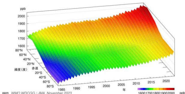
左図と同様。ただしメタン濃度
