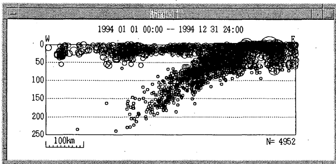
第8図 断面図1の表示例
