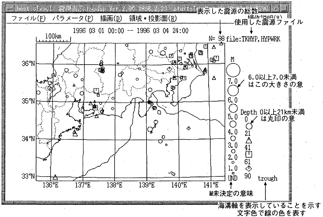
第5図 震央分布図の表示例
