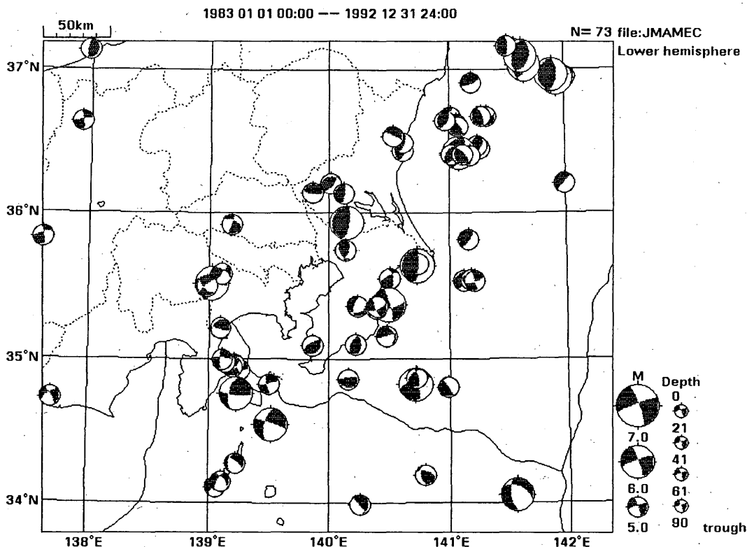
第19図 メカニズム (震源球) の表示例
