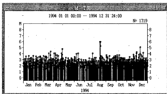
第10図 MT図の表示例
