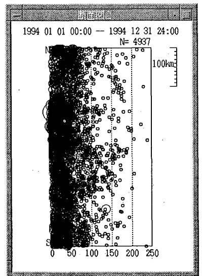
第9図 断面図2の表示例
