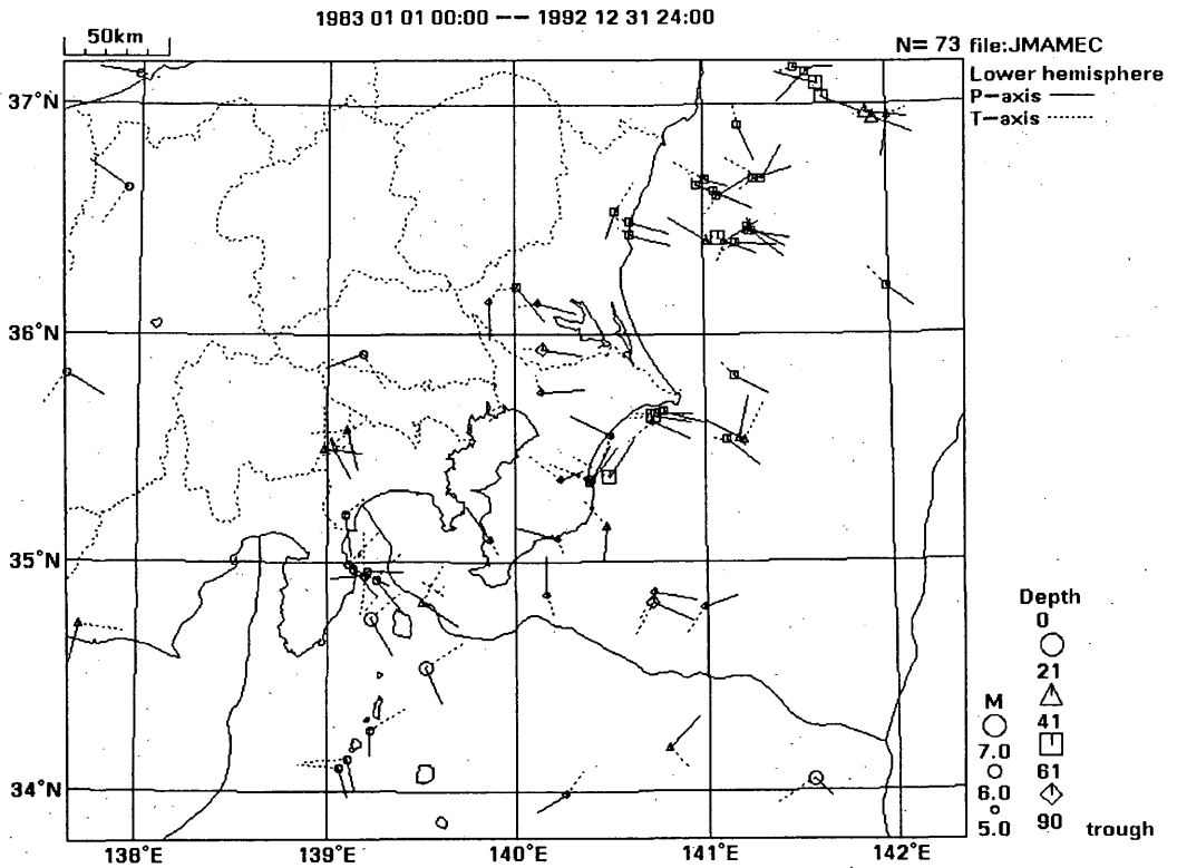
第20図 メカニズム(P,T軸)の表示例
