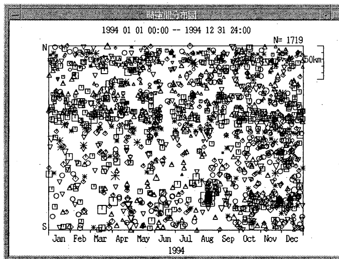
第11図 時空間分布図の表示例
