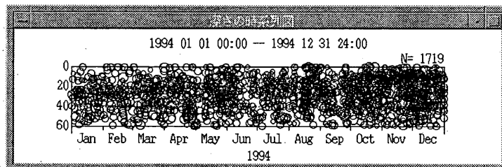
第12図 深さの時系列図の表示例
