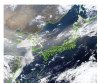
黄砂の情報
