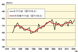
全天日射量の経年変化
