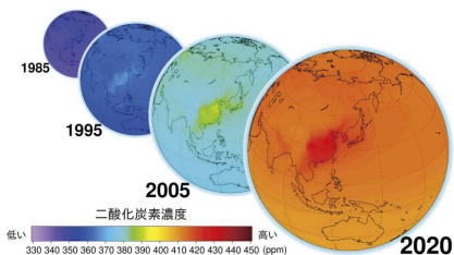
世界の二酸化炭素濃度の変化
