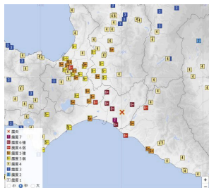
観測された震度の分布図
