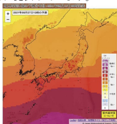
晴天時の UV インデックス
