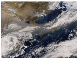
ひまわり黄砂監視画像
