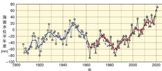
日本沿岸の海面水位変化（1906 年～2021 年）
