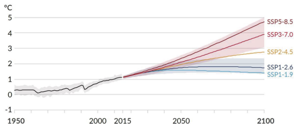
図：1850～1900年を基準とする世界平均気温の変化。
