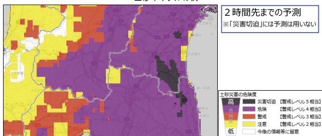
土砂キキクルの例
