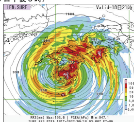
局地モデルによる予測結果
