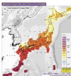
天気分布予報を用いて天気を考慮した UV インデックス
