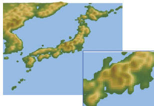
GSM (格子間隔: 約 13km) の地形
