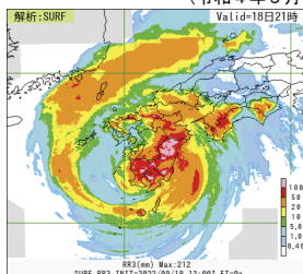
解析雨量
