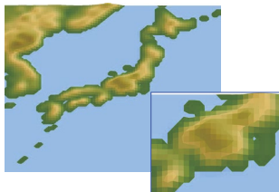
GEPS (格子間隔: 約 27km) の地形
