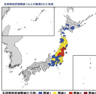
長周期地震動階級1以上が観測された地域 （「長周期地震動の観測結果」より） （令和4年3月16日23時36分の福島県沖の地震、M7.4）
