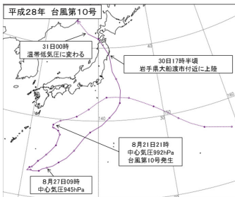
台風経路図
