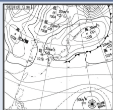
速報天気図
