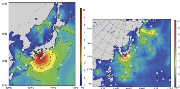
2018 年 9 月 4 日 9 時の沿岸波浪図（左）及び外洋波浪図（右）
