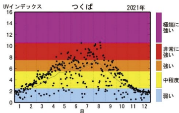
日最大 UV インデックスの季節変化 (実線は 1990～2020 年までの累年平均、丸印は 2021 年)
