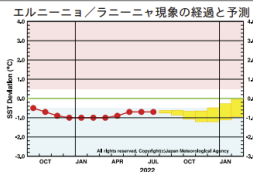
エルニーニョ監視速報(冒頭部分)
