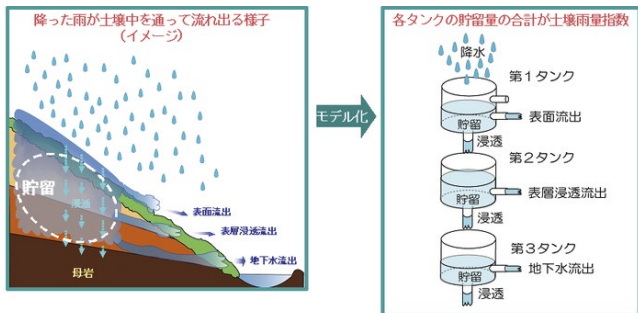
土壌雨量指数のイメージ
