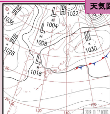
日本域地上天気図
