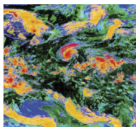
雲の高度の情報
