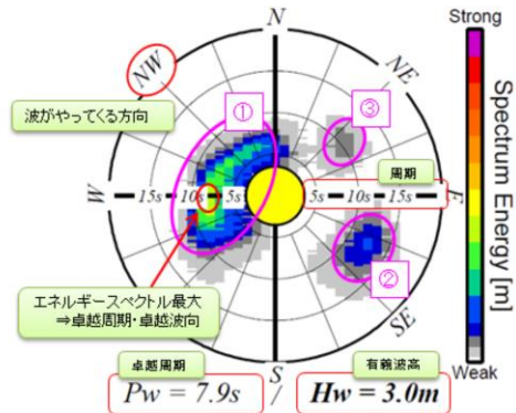
波浪の二次元スペクトル(気象庁仕様)
