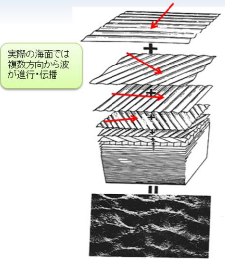
二次元スペクトルの概念図 (Pierson et al. 1955)
