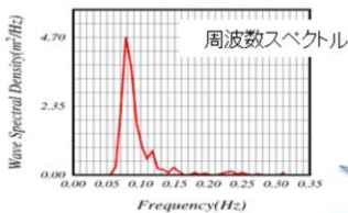
スペクトルの求め方
