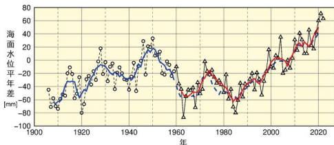
日本沿岸の海面水位変化（1906年～2022年）
