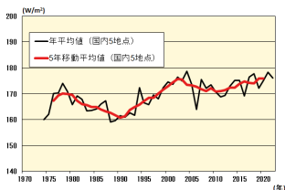
全日射量の経年変化
