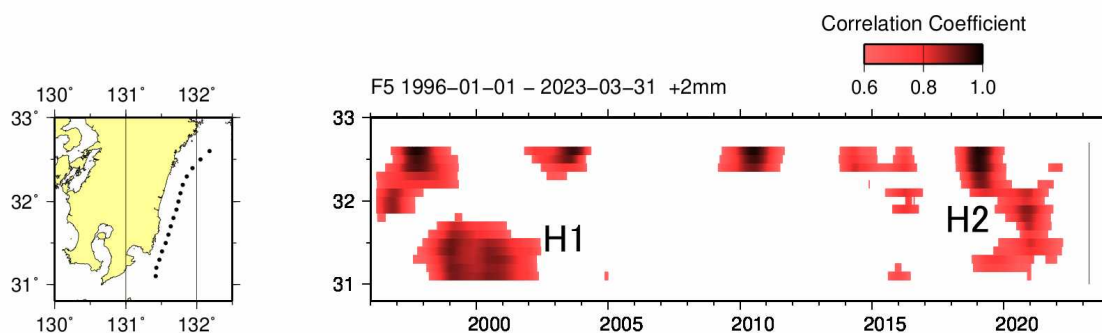
第1図 長期的スロースリップ客観検知図（1996年から2023年3月）
