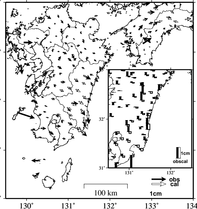
観測値（黒）と計算値（白）の比較 (2022/7/1-2023/4/6)
