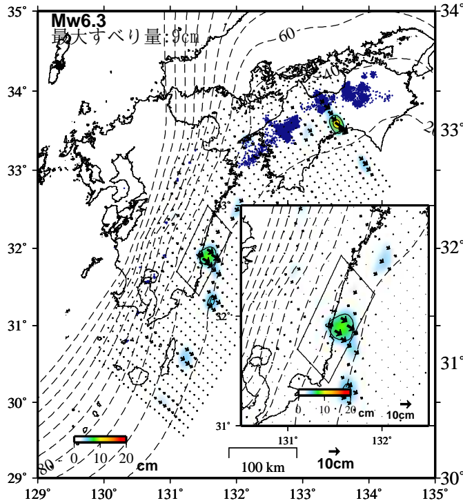
推定すべり分布 (2022/7/1-2023/4/6)
