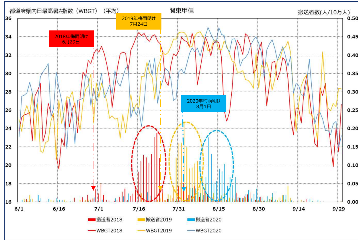
2018~2020年の関東甲信地方での日最高暑さ指数(WBGT)と日ごとの重篤な搬送者数の推移
