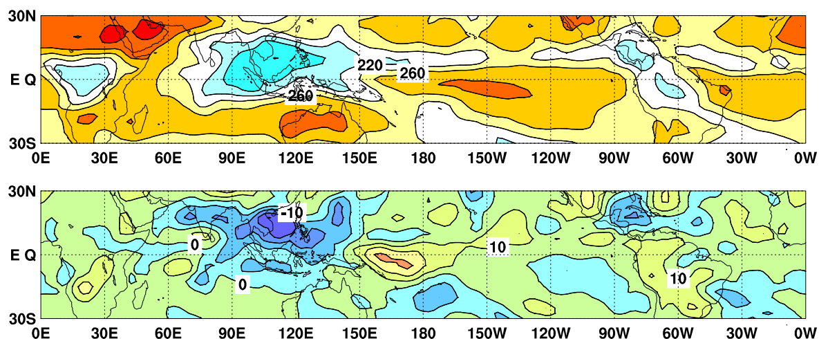
図 9 外向き長波放射量 (OLR) (上) 及び年偏差 (下) の分布図 (2020 年 10 月)
