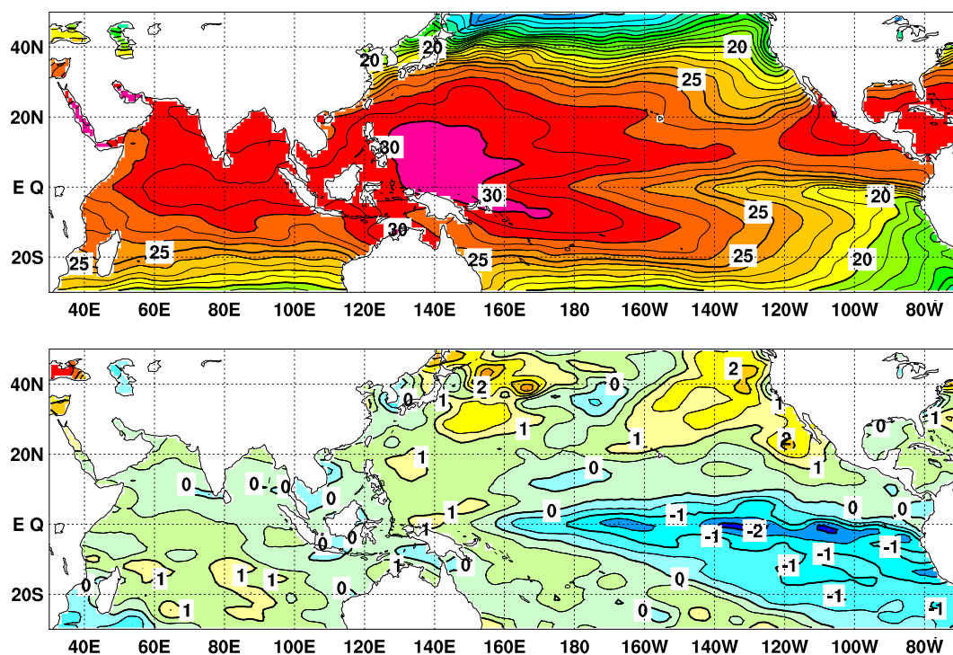
図4 2020年10月の海面水温図（上）及び平年偏差図（下）
