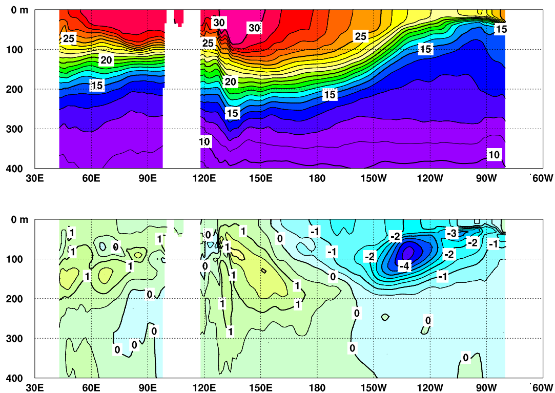
図5 2020年10月のインド洋から太平洋の赤道に沿った水温（上）及び平年偏差（下）の断面図
