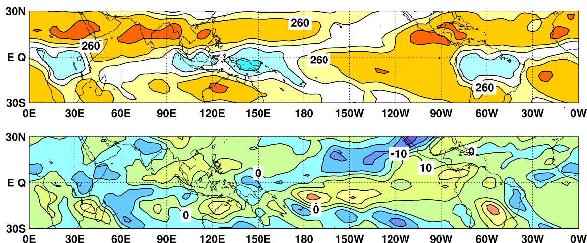
図 9 外向き長波放射量 (OLR) (上) 及び年偏差 (下) の分布図 (2020 年 3 月)
