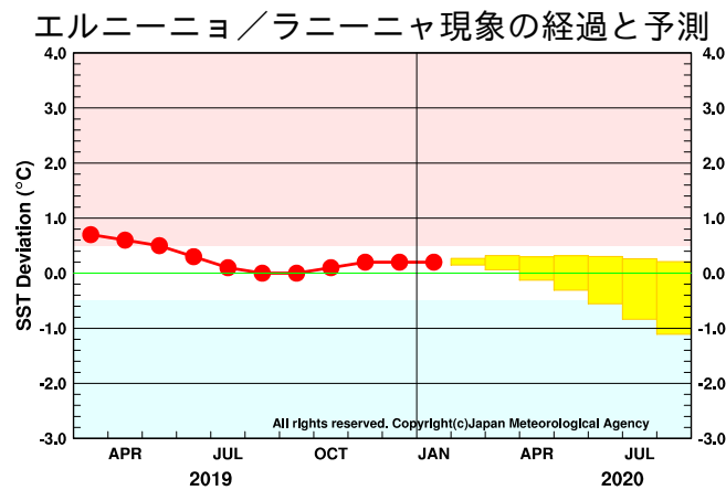
図 1 エルニーニョ監視海域の海面水温の基準値との差の 5 か月移動平均値 1 月までの経過（観測値）を折れ線グラフで、エルニーニョ予測モデルによる予測結果（70%の確率で入ると予想される範囲）をボックスで示している。指数が赤／青の範囲に入っている期間がエルニーニョ／ラニーニャ現象の発生期間である。エルニーニョ監視海域の海面水温の基準値はその年の前年までの 30 年間の各月の平均値。
