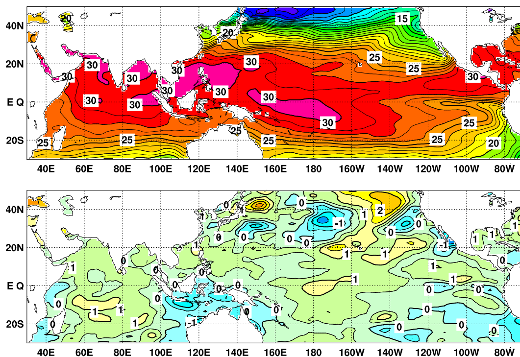
図4 2019年6月の海面水温図（上）及び平年偏差図（下）
