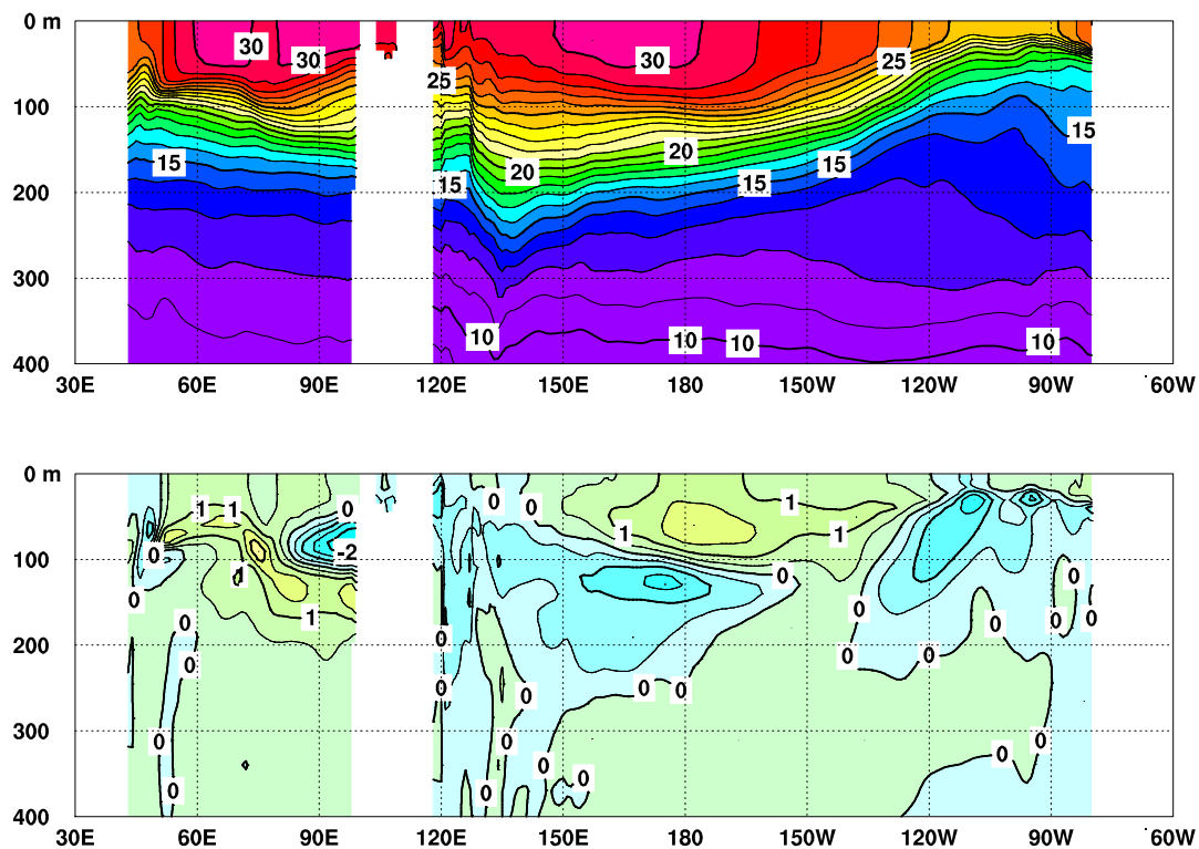
図5 2019年6月のインド洋から太平洋の赤道に沿った水温（上）及び平年偏差（下）の断面図
