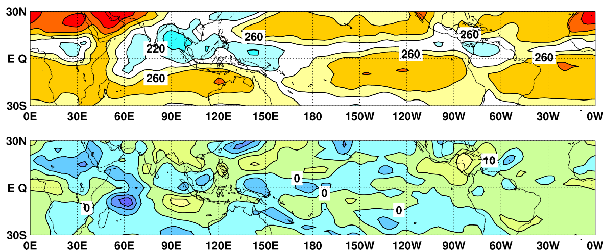
図 9 外向き長波放射量 (OLR) (上) 及び年偏差 (下) の分布図 (2019 年 6 月)
