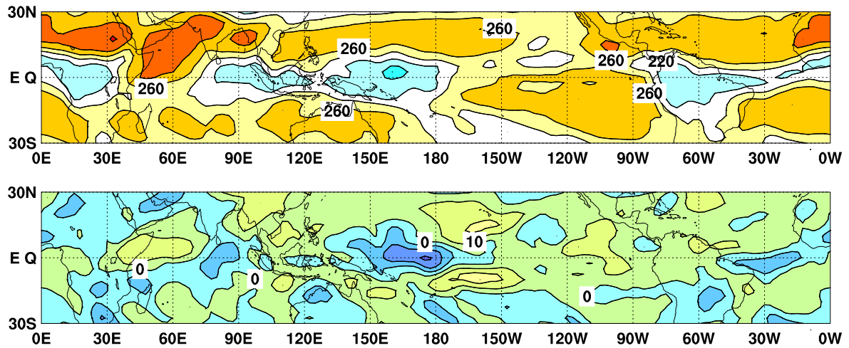
図 9 外向き長波放射量 (OLR) (上) 及び年偏差 (下) の分布図 (2019 年 4 月)
