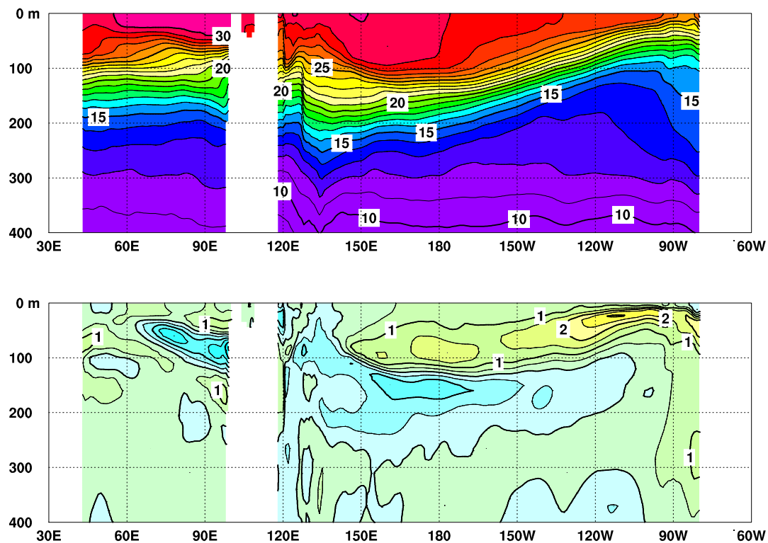
図5 2019年4月のインド洋から太平洋の赤道に沿った水温（上）及び平年偏差（下）の断面図
