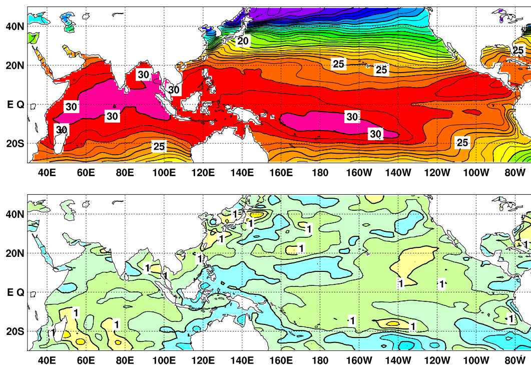
図4 2019年4月の海面水温図（上）及び平年偏差図（下）
