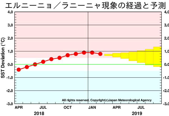
図 1 エルニーニョ監視海域の海面水温の基準値との差の 5 か月移動平均値 2 月までの経過（観測値）を折れ線グラフで、エルニーニョ予測モデルによる予測結果（70%の確率で入ると予想される範囲）をボックスで示している。指数が赤／青の範囲に入っている期間がエルニーニョ／ラニーニャ現象の発生期間である。エルニーニョ監視海域の海面水温の基準値はその年の前年までの 30 年間の各月の平均値。
