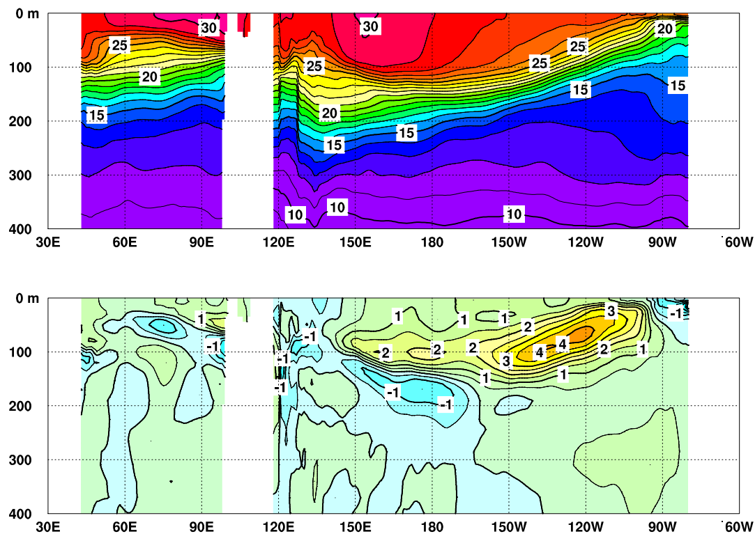
図5 2019年3月のインド洋から太平洋の赤道に沿った水温（上）及び平年偏差（下）の断面図
