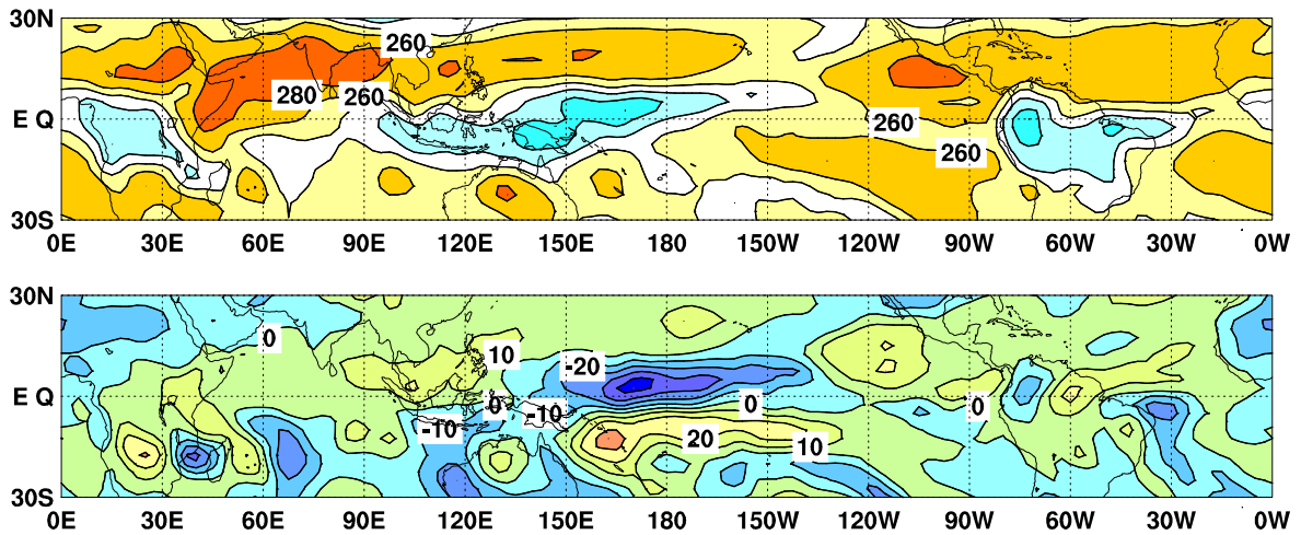
図9 外向き長波放射量 (OLR) (上) 及び平年偏差 (下) の分布図 (2019年3月)
