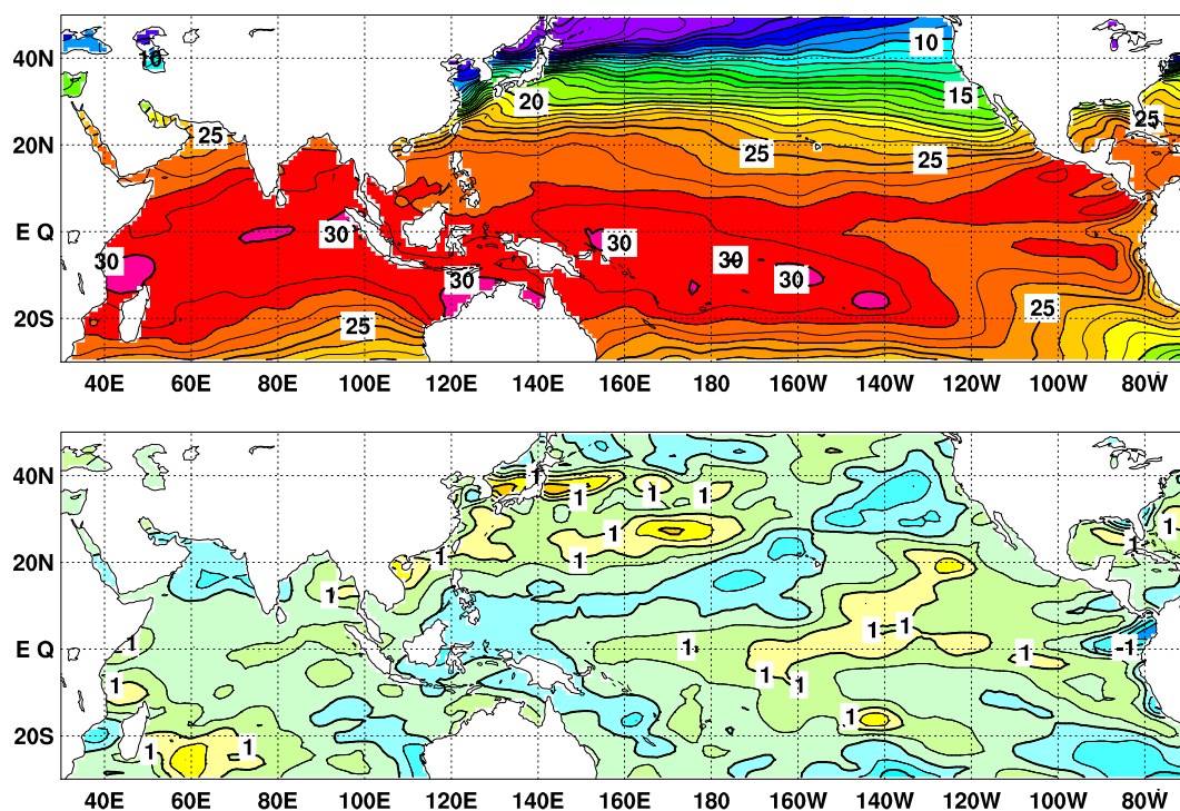
図4 2019年3月の海面水温図（上）及び平年偏差図（下）
