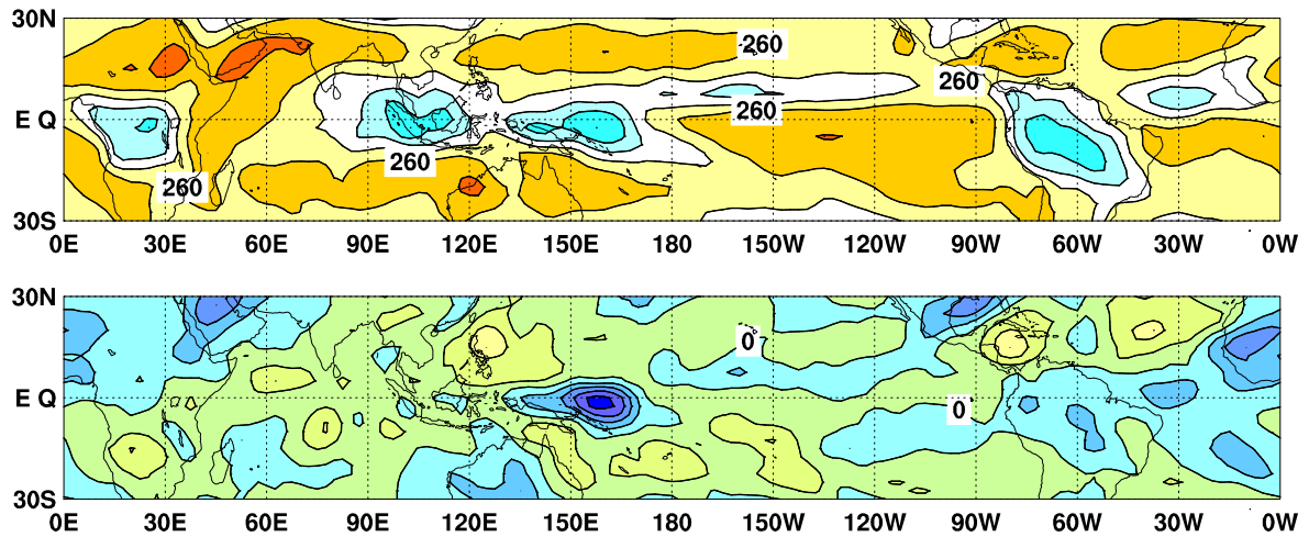
図 9 外向き長波放射量 (OLR) (上) 及び年平均偏差 (下) の分布図 (2018 年 11 月)
