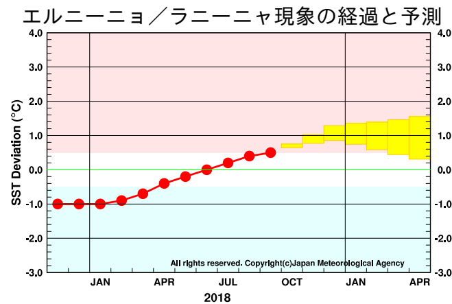
図 1 エルニーニョ監視海域の海面水温の基準値との差の 5 か月移動平均値 9 月までの経過（観測値）を折れ線グラフで、エルニーニョ予測モデルによる予測結果（70%の確率で入ると予想される範囲）をボックスで示している。指数が赤／青の範囲に入っている期間がエルニーニョ／ラニーニャ現象の発生期間である。エルニーニョ監視海域の海面水温の基準値はその年の前年までの 30 年間の各月の平均値。
