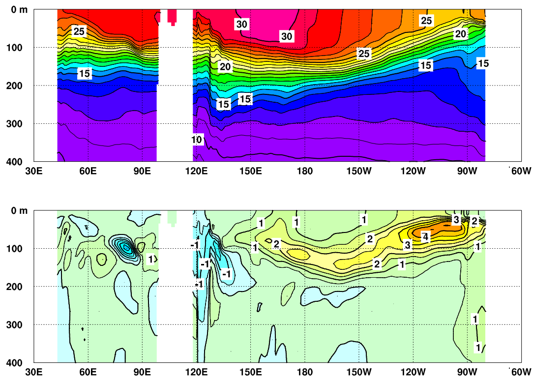
図5 2018年11月のインド洋から太平洋の赤道に沿った水温（上）及び平年偏差（下）の断面図
