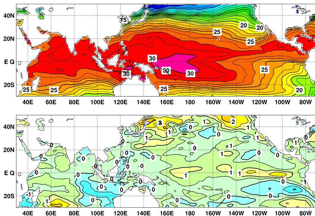
図4 2018年11月の海面水温図（上）及び平年偏差図（下）
