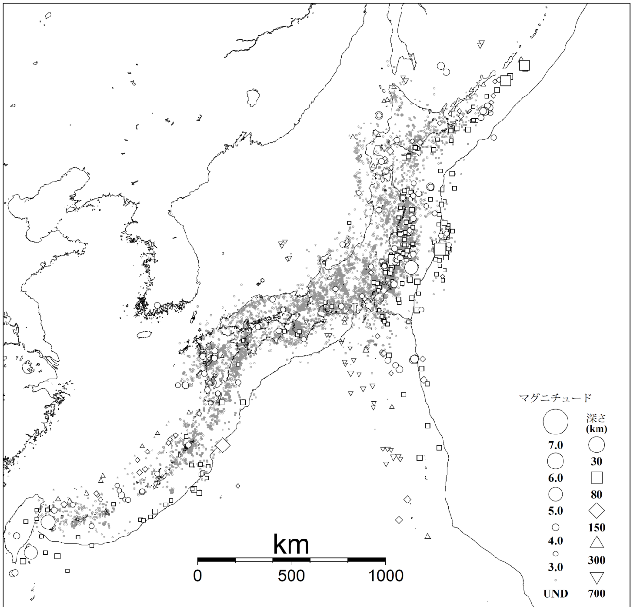
図3 気象庁が震源を決定した日本付近の平成 29 年 10 月の地震の震央分布 (M3.0 以上の地震については白抜きで示す)
