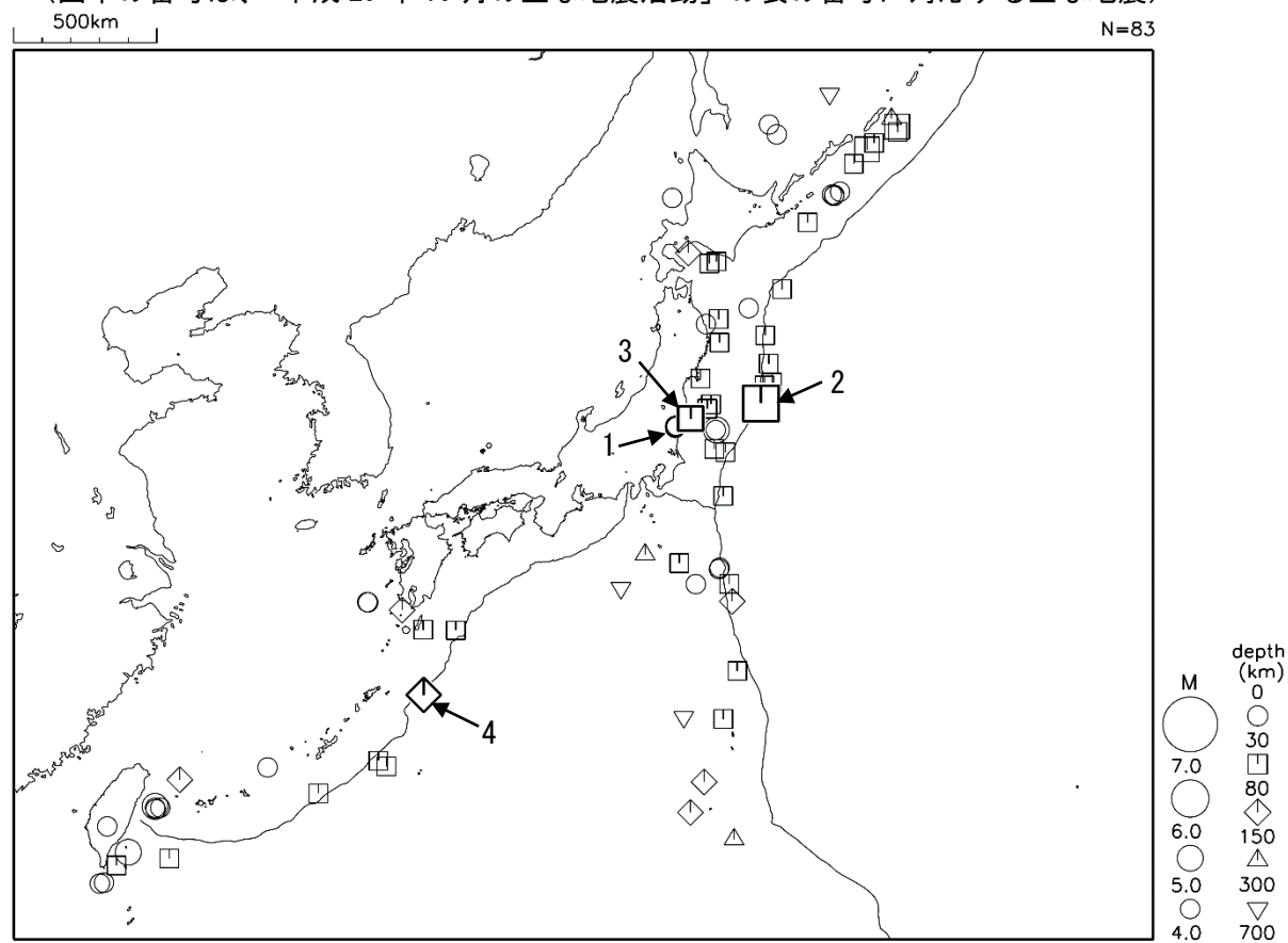
図 2 平成 29 年 10 月に発生した M4.0 以上の地震 (図中の番号は、「平成 29 年 10 月の主な地震活動」の表の番号に対応する主な地震)
