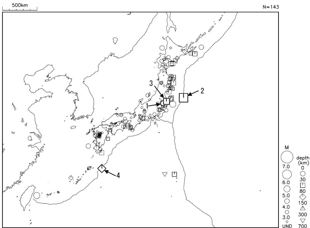
図 1 平成 29 年 10 月に震度 1 以上を観測した地震 (図中の番号は、「平成 29 年 10 月の主な地震活動」の表の番号に対応する主な地震)
