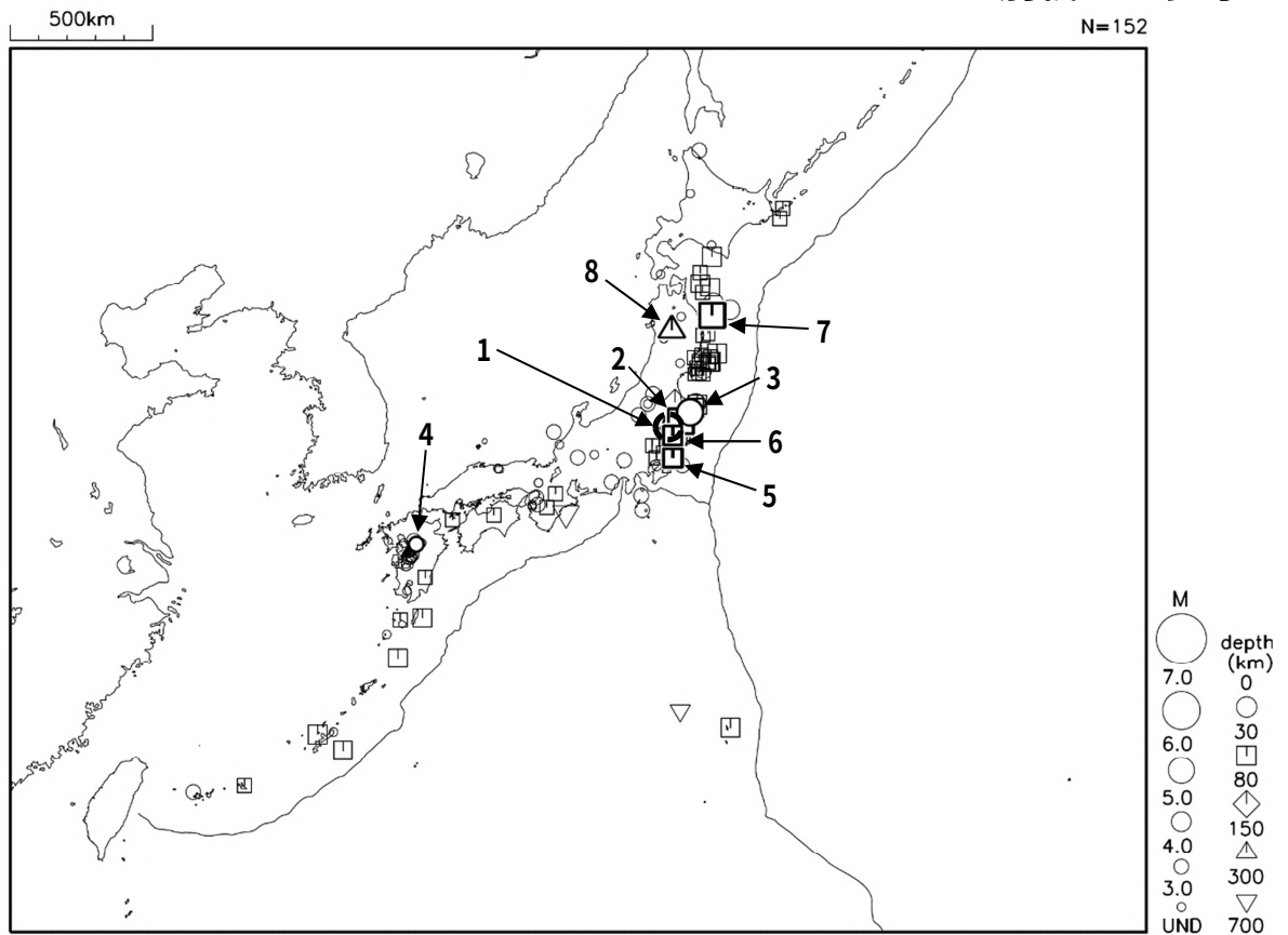
図1 平成29年1月に震度1以上を観測した地震 (図中の番号は、「平成29年1月の主な地震活動」の表の番号に対応する主な地震)
