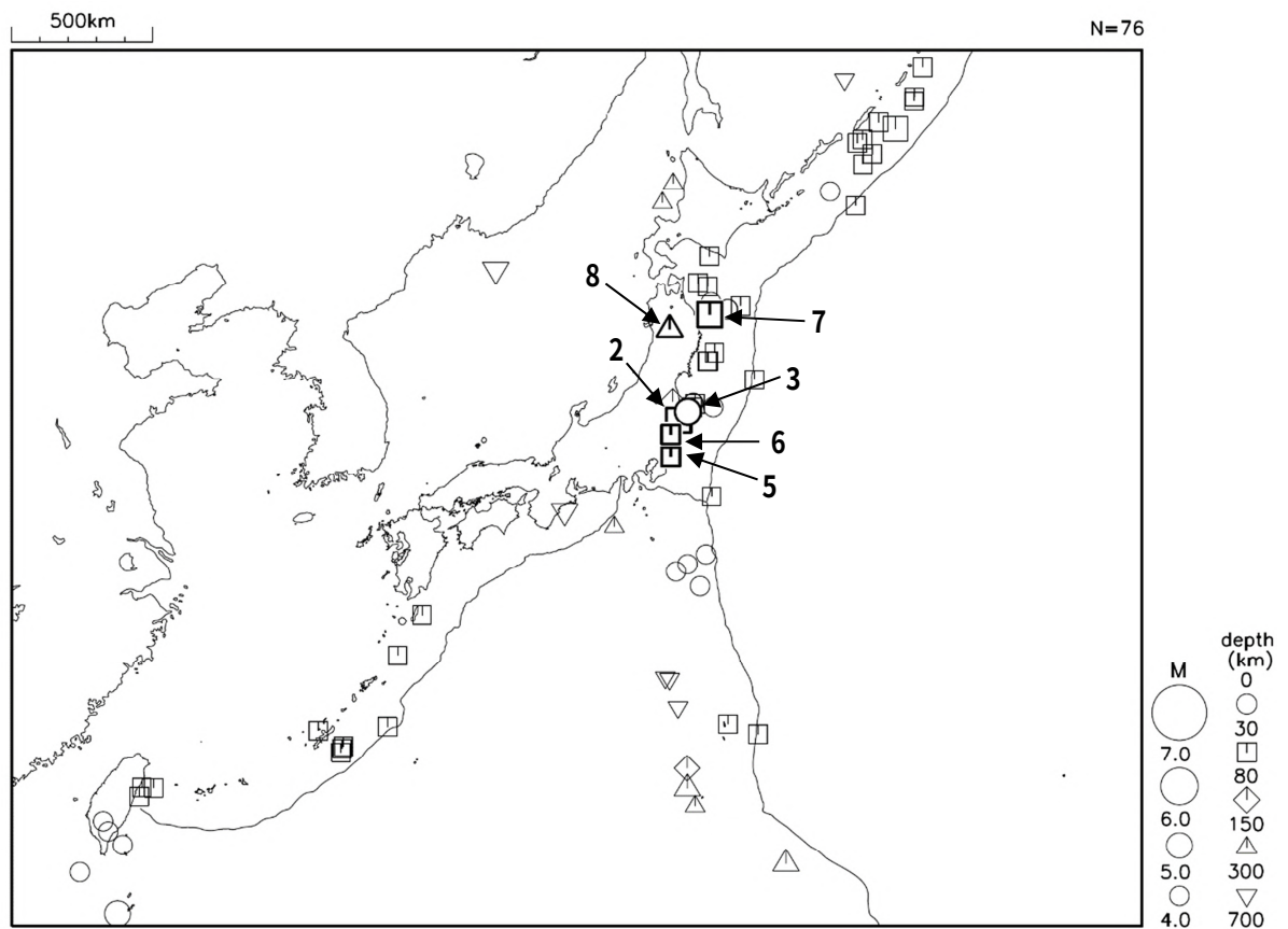
図2 平成29年1月に発生したM4.0以上の地震 (図中の番号は、「平成29年1月の主な地震活動」の表の番号に対応する主な地震)
