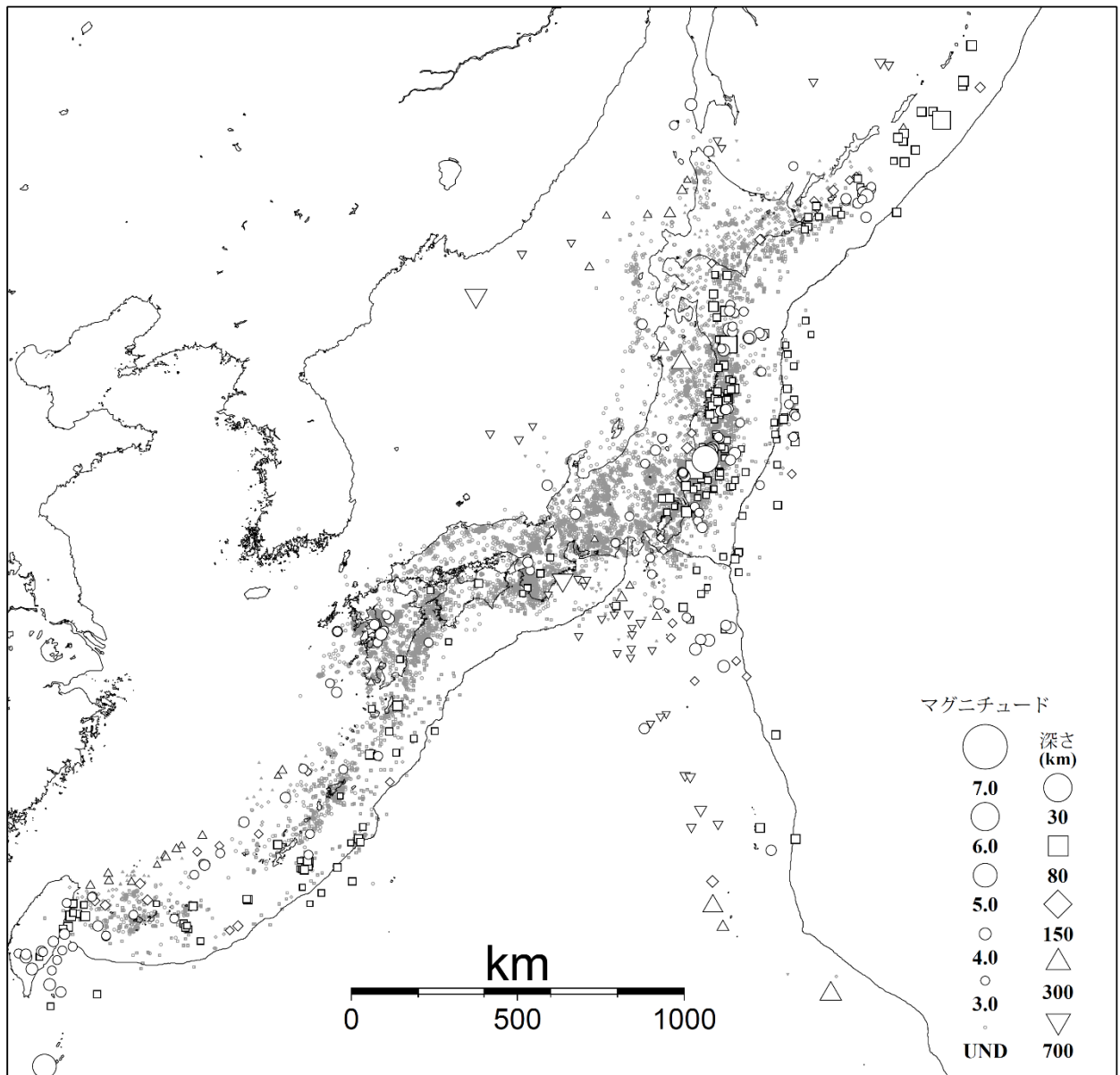
図3 気象庁が震源を決定した日本付近の平成 29 年 1 月の地震の震央分布 (M3.0 以上の地震については白抜きで示す)
