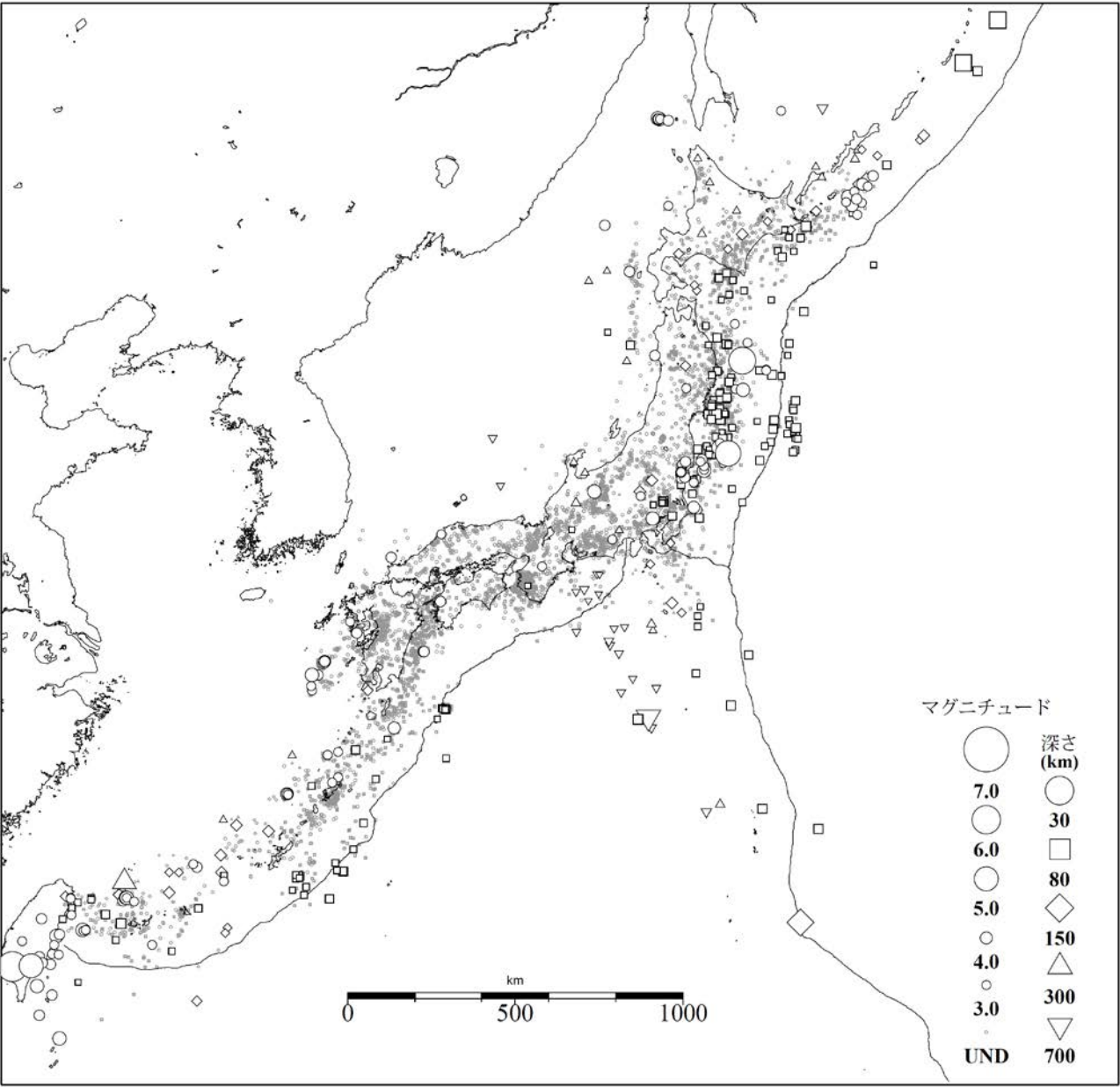
図3 気象庁が震源を決定した日本付近の平成28年2月の地震の震央分布 (M3.0以上の地震については白抜きで示す)
