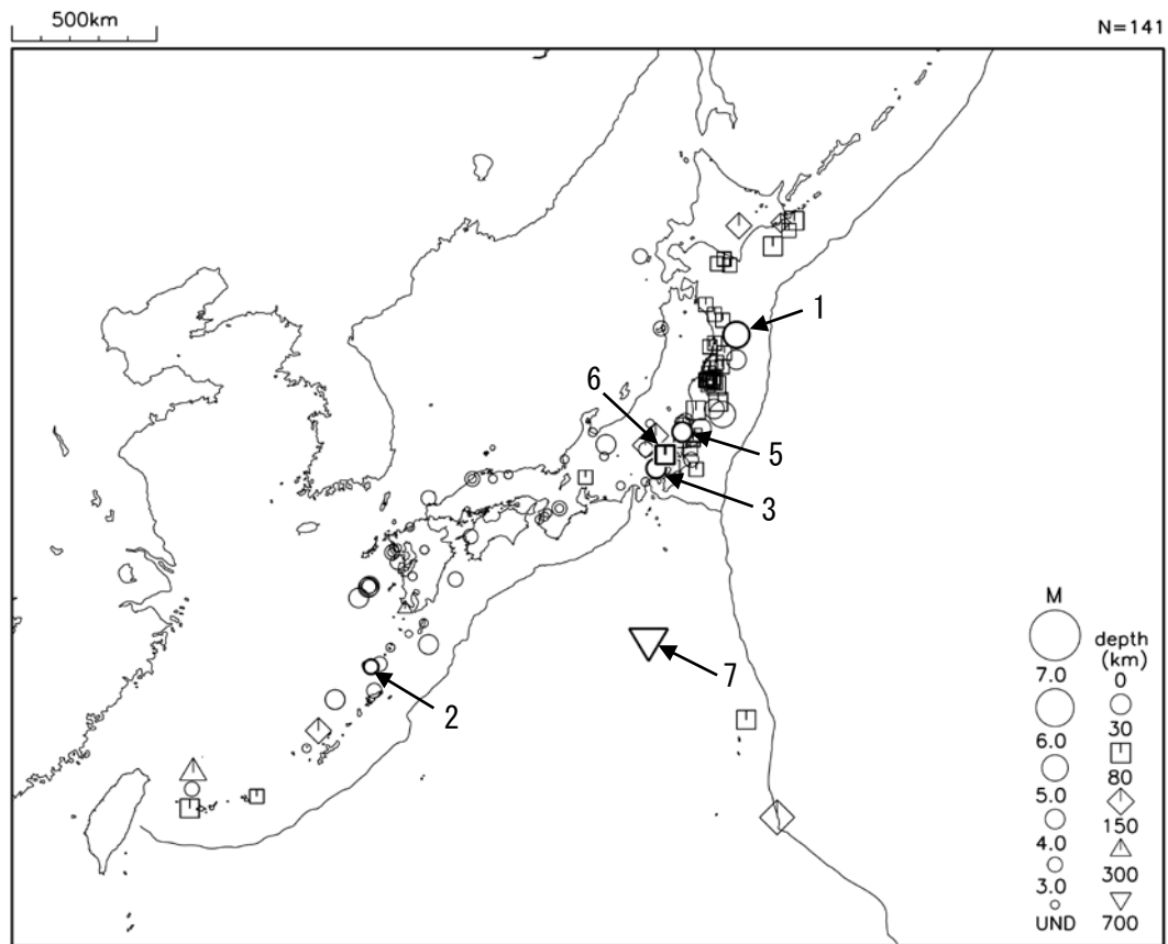
図 1 平成 28 年 2 月に震度 1 以上を観測した地震 (図中の番号は、「平成 28 年 2 月の主な地震活動」の表の番号に対応する主な地震)
