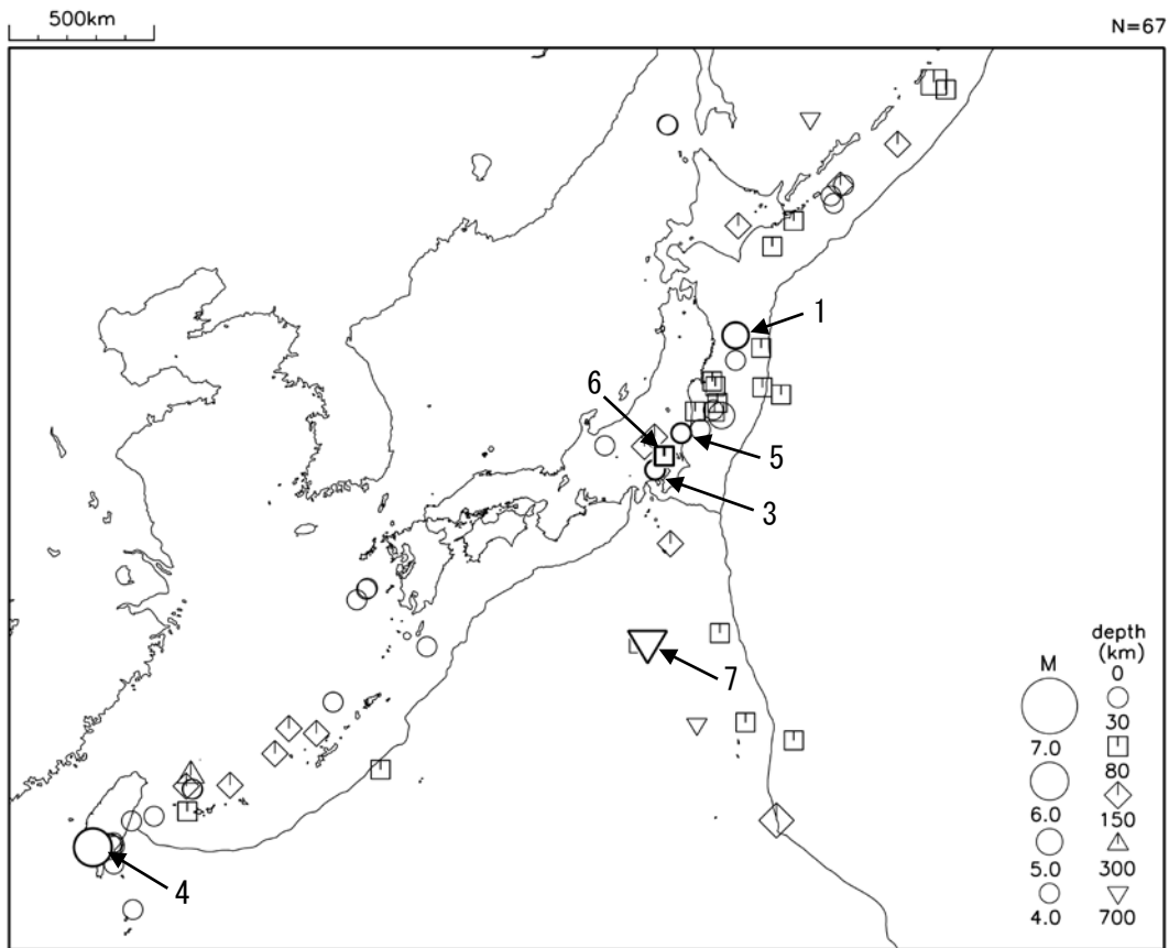
図 2 平成 28 年 2 月に発生した M4.0 以上の地震 (図中の番号は、「平成 28 年 2 月の主な地震活動」の表の番号に対応する主な地震)
