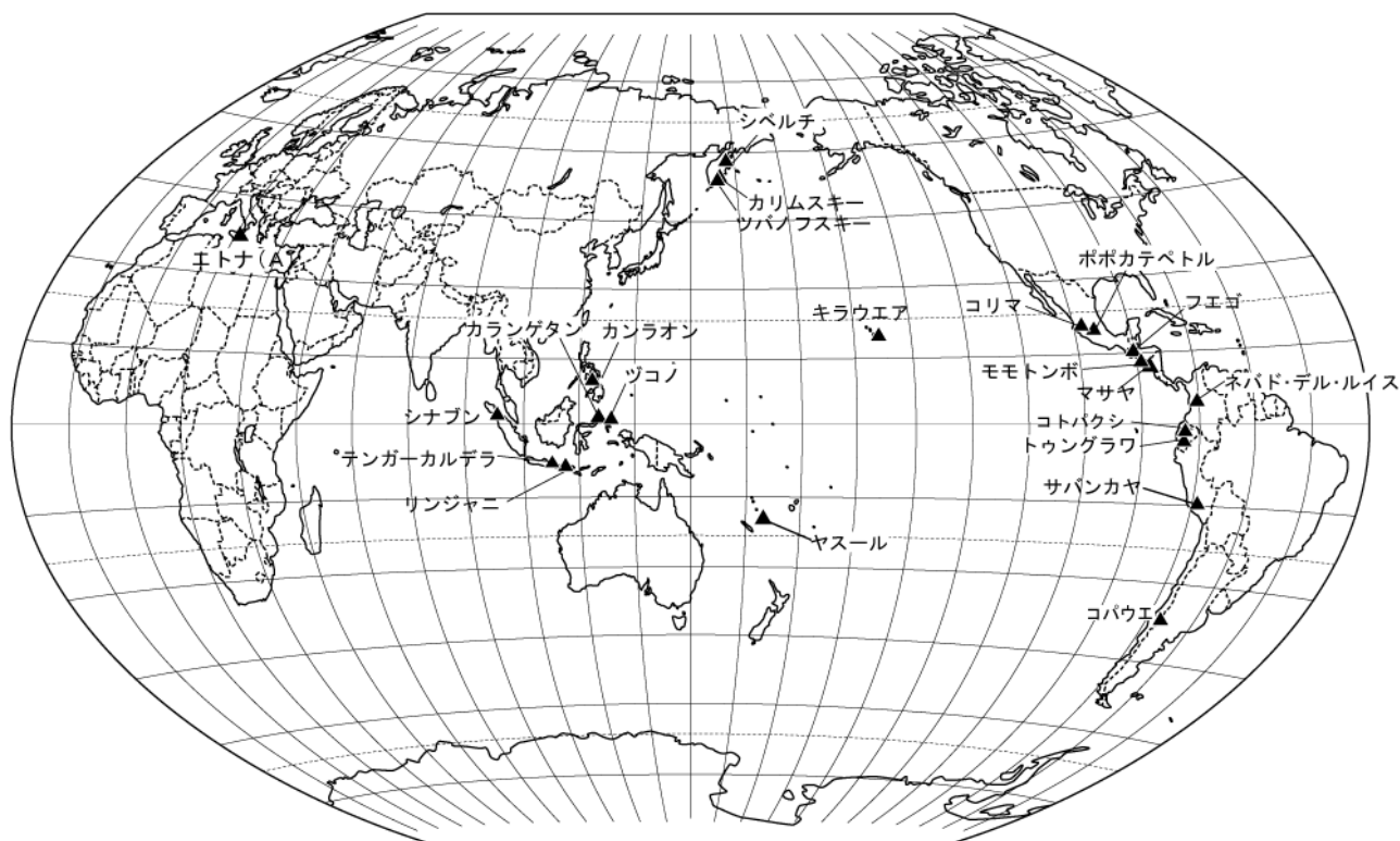
図 平成 27 年（2015 年）12 月に噴火した主な火山（日本を除く）*
