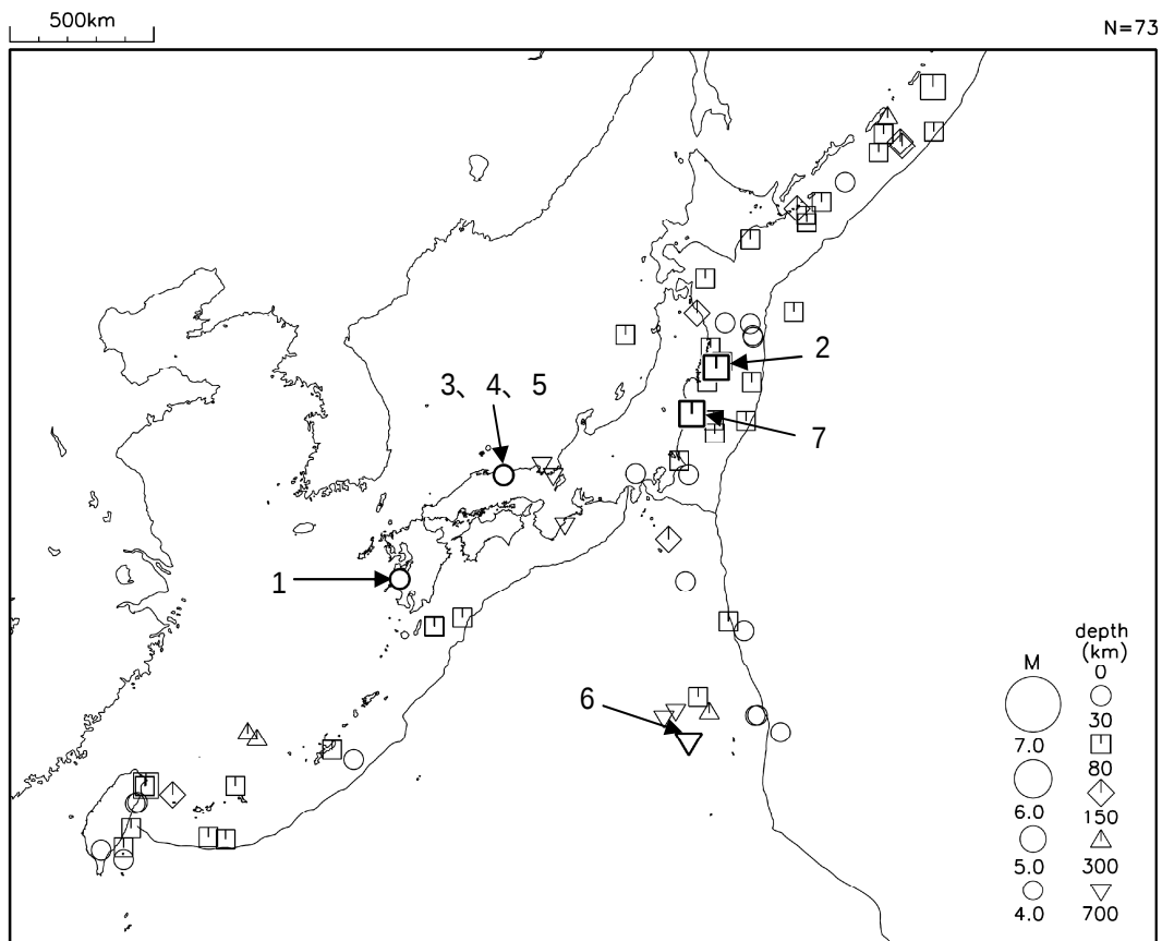
図2 平成 27 年 10 月に発生した M4.0 以上の地震 ( 図中の番号は、「平成 27 年 10 月の主な地震活動」の表の番号に対応する主な地震 )
