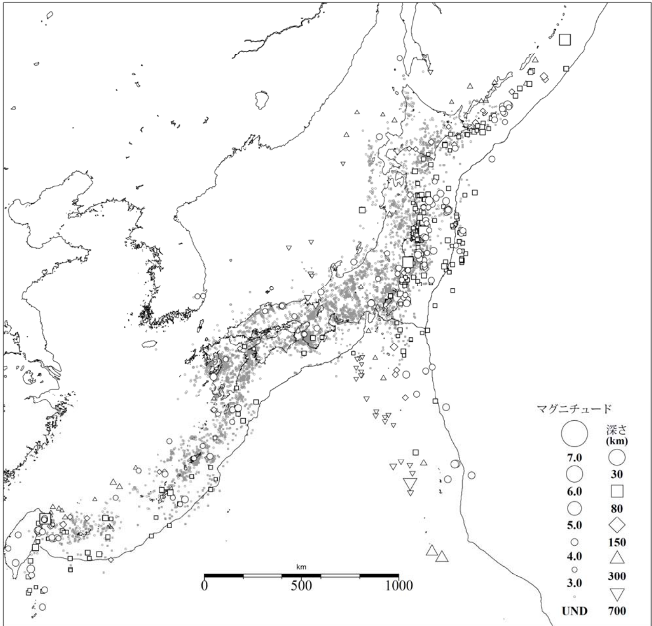
図3 気象庁が震源を決定した日本付近の平成27年10月の地震の震央分布 (M3.0以上の地震については白抜きで示す)
