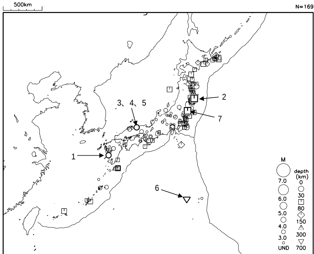
図1 平成 27 年 10 月に震度 1 以上を観測した地震 ( 図中の番号は、「平成 27 年 10 月の主な地震活動」の表の番号に対応する主な地震 )
