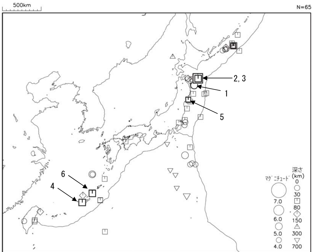
図2 平成26年10月に発生したM4.0以上の地震 (図中の番号は、「平成26年10月の主な地震活動」の表の番号に対応する主な地震)
