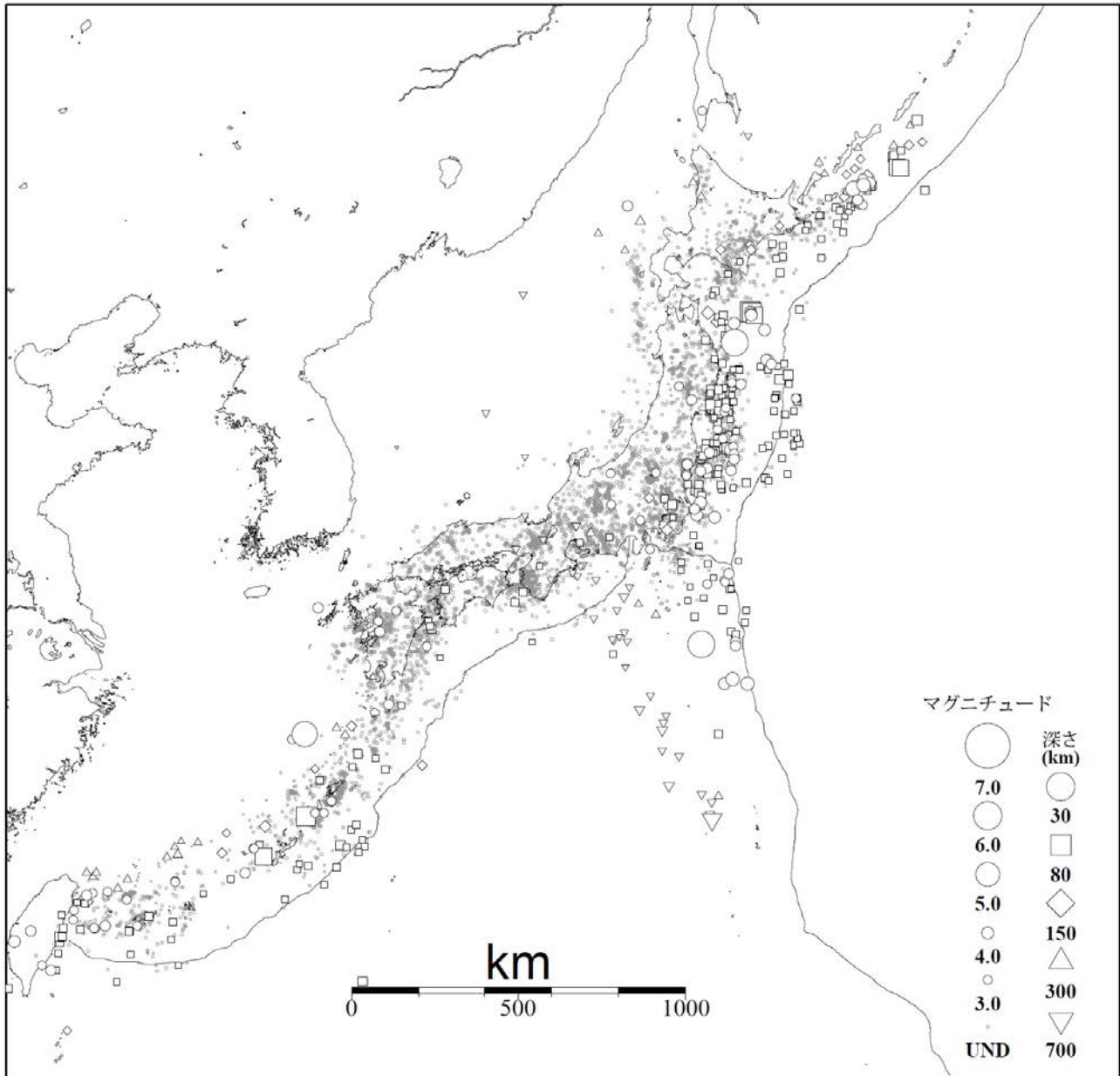
図3 気象庁が震源を決定した日本付近の平成26年10月の地震の震央分布 (M3.0以上の地震については白抜きで示す)
