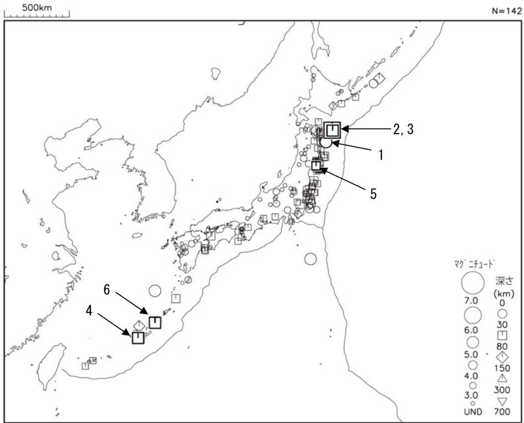
図1 平成26年10月に震度1以上を観測した地震 (図中の番号は、「平成26年10月の主な地震活動」の表の番号に対応する主な地震)
