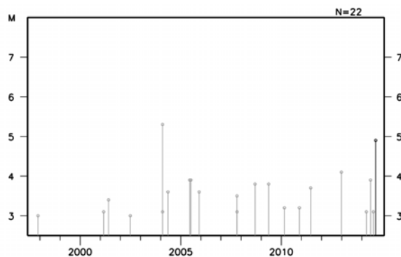
領域b内のM-T図 ( M \geq 3.0 )
