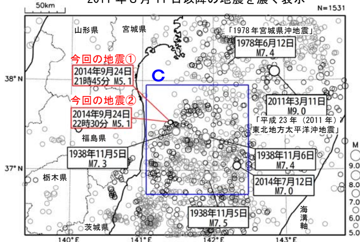
震央分布図 (1923年1月1日～2014年9月30日、 深さ0～150km、 M \geq 5.0 )
