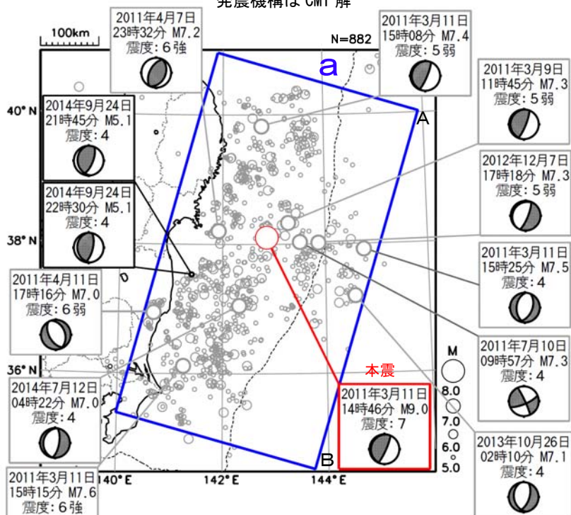
震央分布図 (2011 年 3 月 1 日～2014 年 9 月 30 日、深さすべて、M ≥ 5.0)
