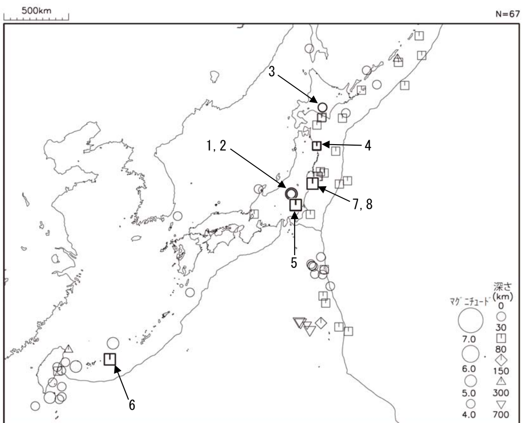
図 2 平成 26 年 9 月に発生した M4.0 以上の地震 (図中の番号は、「平成 26 年 9 月の主な地震活動」の表の番号に対応する主な地震)
