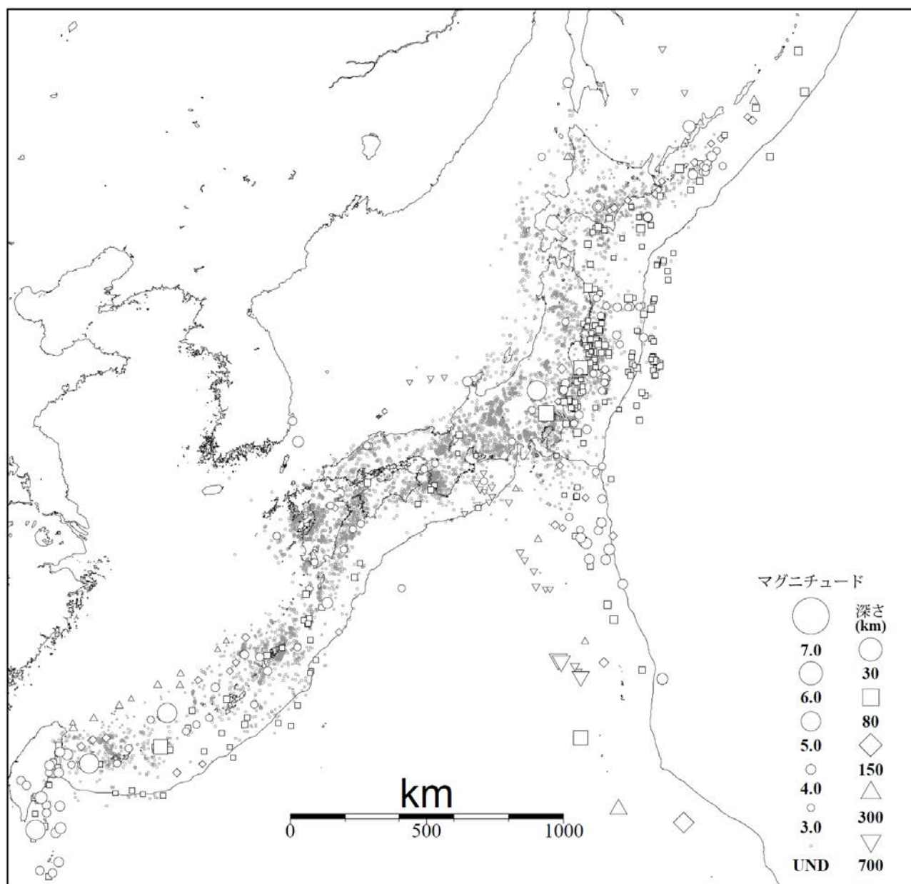
図3 気象庁が震源を決定した日本付近の平成26年9月の地震の震央分布 (M3.0以上の地震については白抜きで示す)
