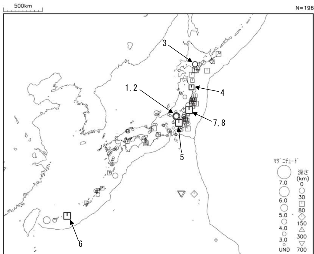
図 1 平成 26 年 9 月に震度 1 以上を観測した地震 (図中の番号は、「平成 26 年 9 月の主な地震活動」の表の番号に対応する主な地震)
