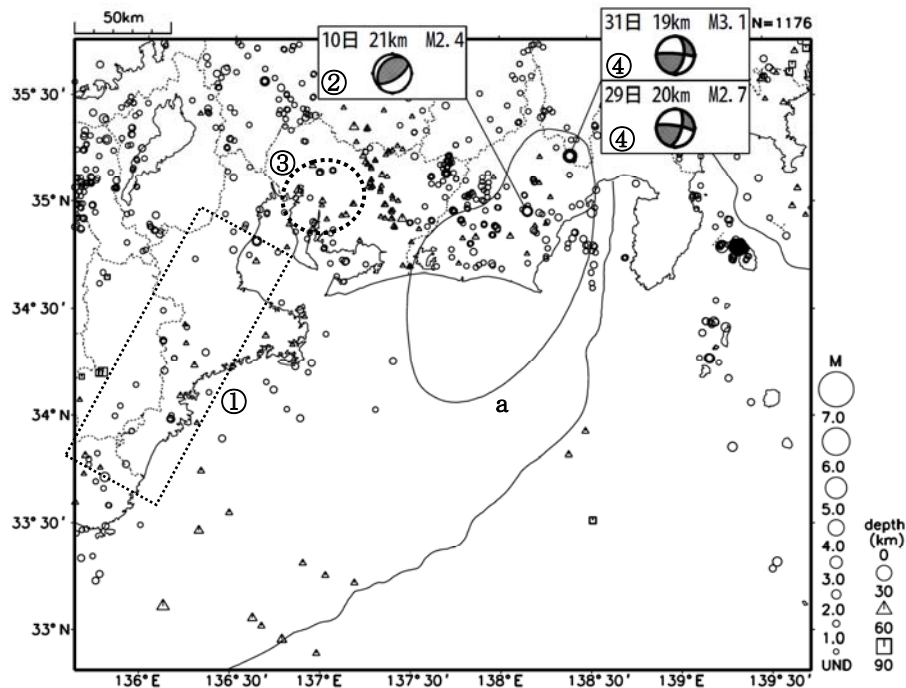
図1 震央分布図（2014年7月1日～31日：深さ0～90km、Mすべて。図中の領域aは東海地震の想定震源域。）
