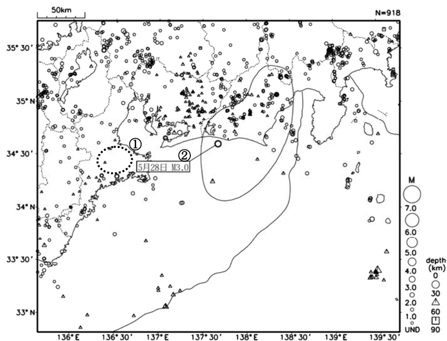
図1 震央分布図(2014年5月1日～31日:深さ0～90km、Mすべて。図中のナス型の領域は東海地震の想定震源域。)
