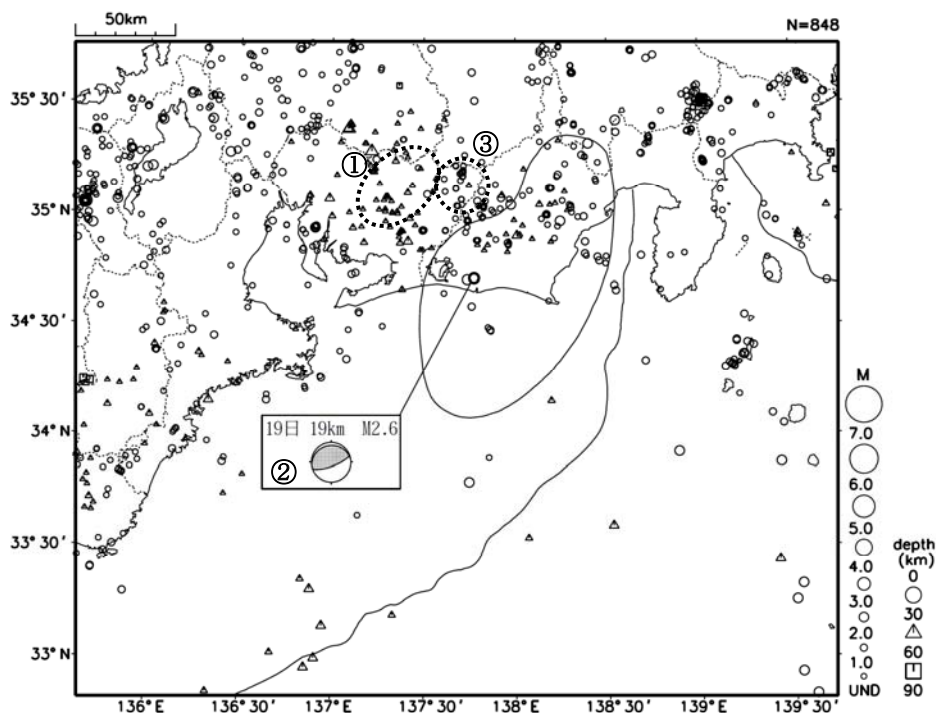
図1 震央分布図(2014年4月1日～30日:深さ0～90km、Mすべて。図中のナス型の領域は東海地震の想定震源域。)
