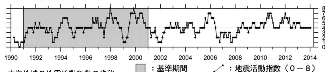
図3 東海地域の地震活動指数の推移
