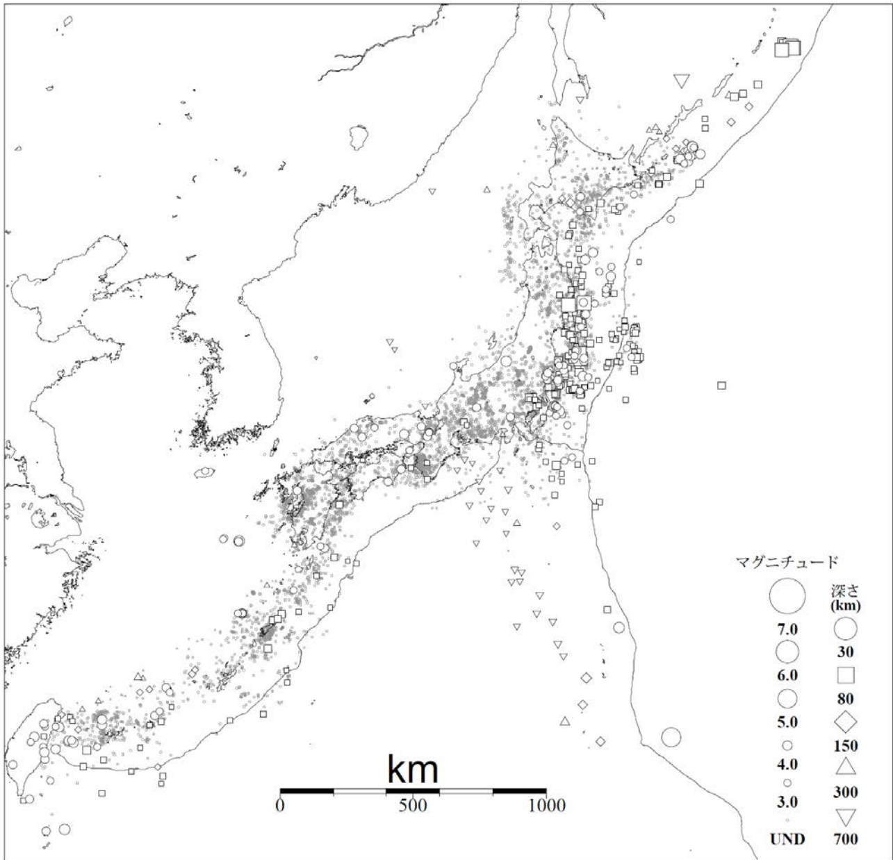
図3 気象庁が震源を決定した日本付近の平成26年4月の地震の震央分布 (M3.0以上の地震については白抜きで示す)
