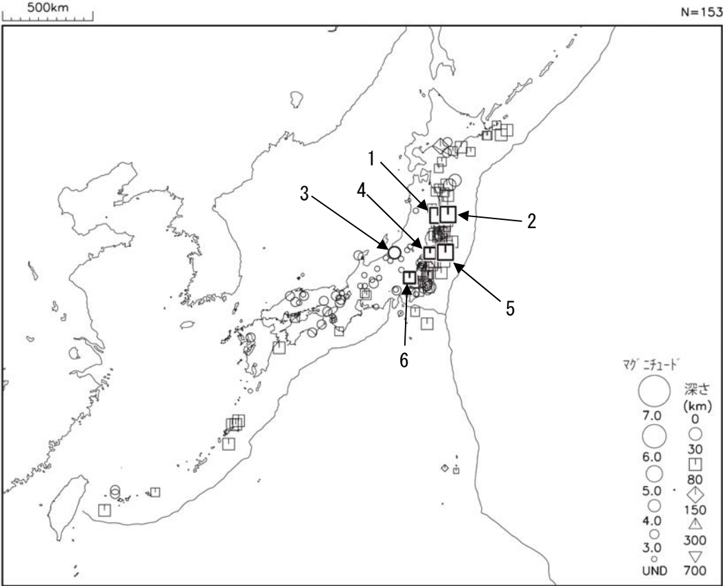
図 1 平成 26 年 4 月に震度 1 以上を観測した地震 (図中の番号は、「平成 26 年 4 月の主な地震活動」の表の番号に対応する主な地震)
