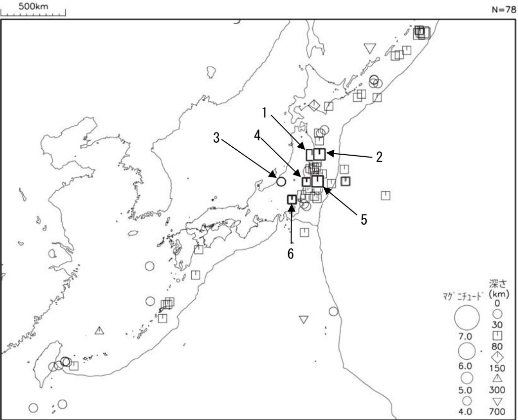
図 2 平成 26 年 4 月に発生した M4.0 以上の地震 (図中の番号は、「平成 26 年 4 月の主な地震活動」の表の番号に対応する主な地震)
