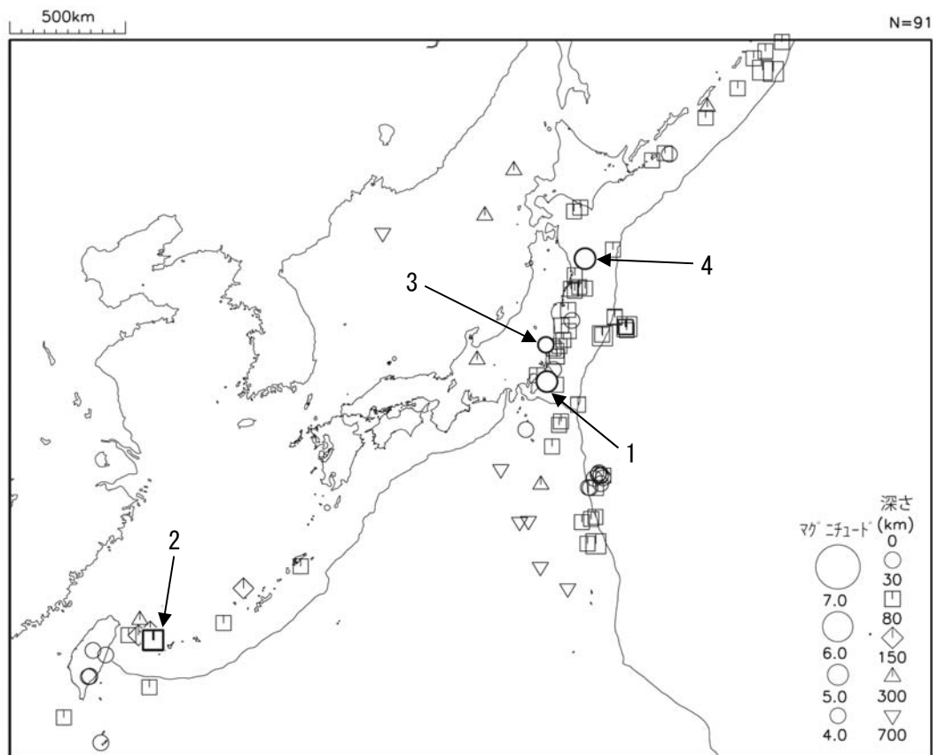
図2 平成26年1月に発生したM4.0以上の地震 (図中の番号は、「平成26年1月の主な地震活動」の表の番号に対応する主な地震)
