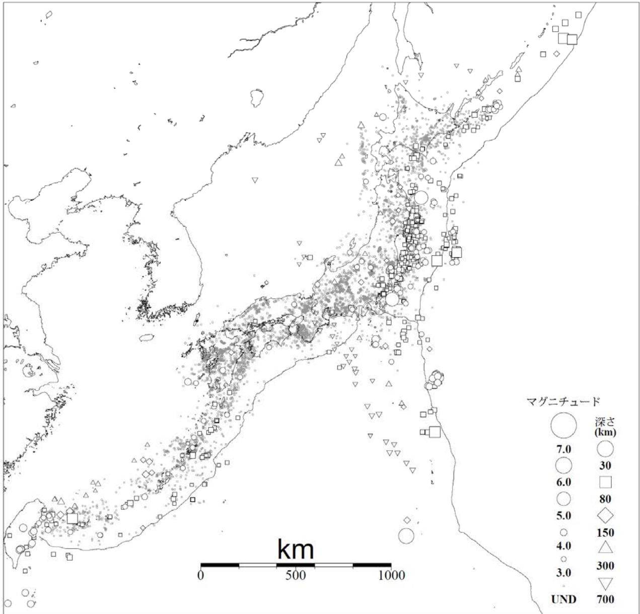
図3 気象庁が震源を決定した日本付近の平成26年1月の地震の震央分布 (M3.0以上の地震については白抜きで示す)
