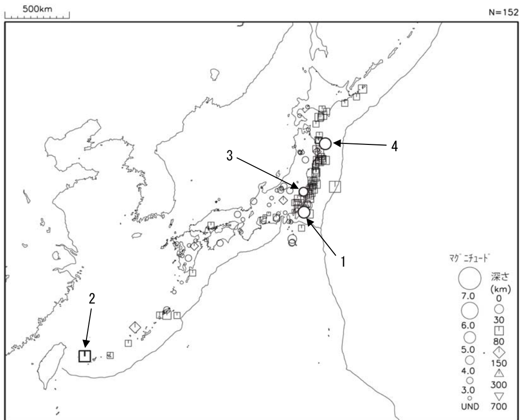
図1 平成26年1月に震度1以上を観測した地震 (図中の番号は、「平成26年1月の主な地震活動」の表の番号に対応する主な地震)
