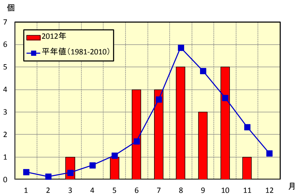
図2 2012年（平成24年）の月別発生数（12月21日現在） 赤：発生数、青：平年値（1981～2010年の30年平均値）
