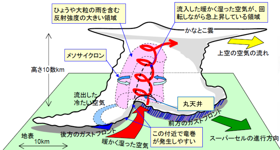
スーパーセルの模式図
