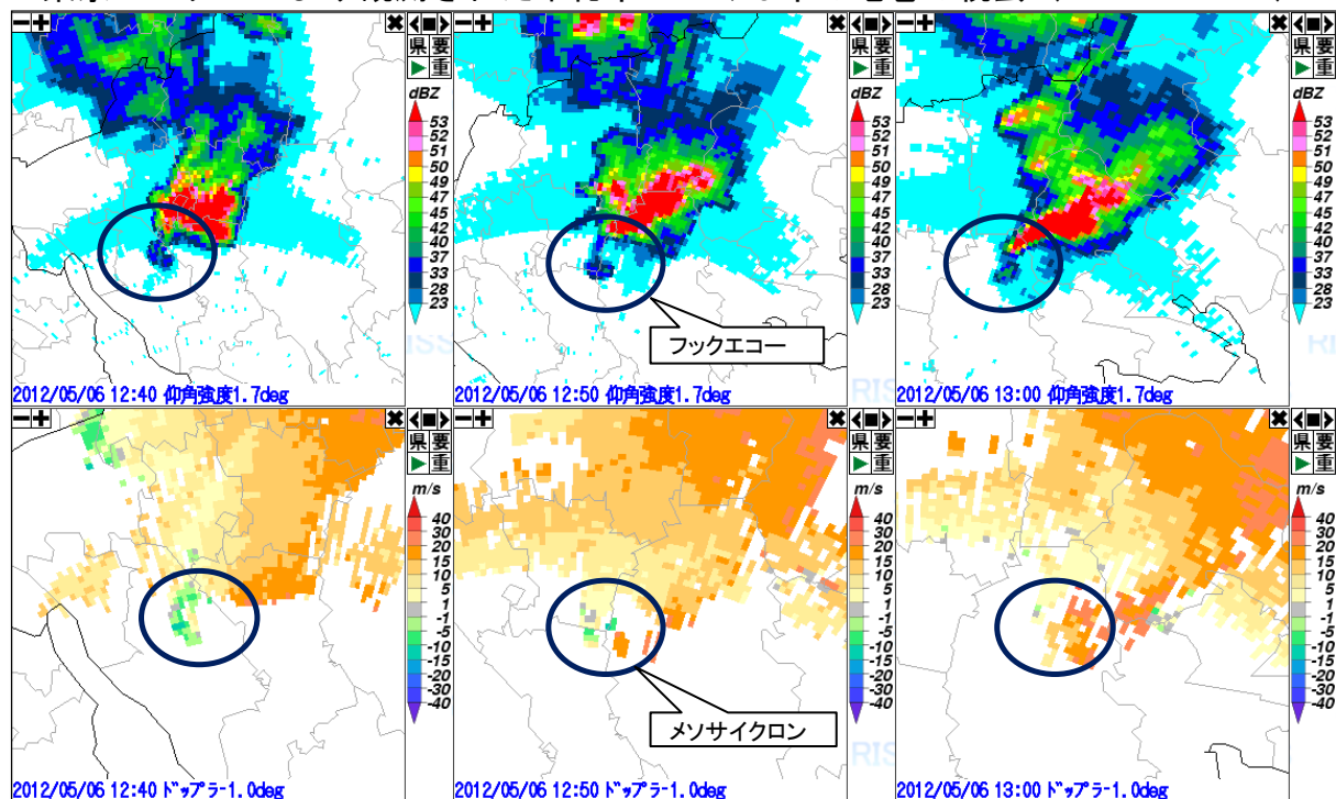
東京レーダーにより観測された常総市～つくば市の竜巻の親雲（12:40～13:00）
