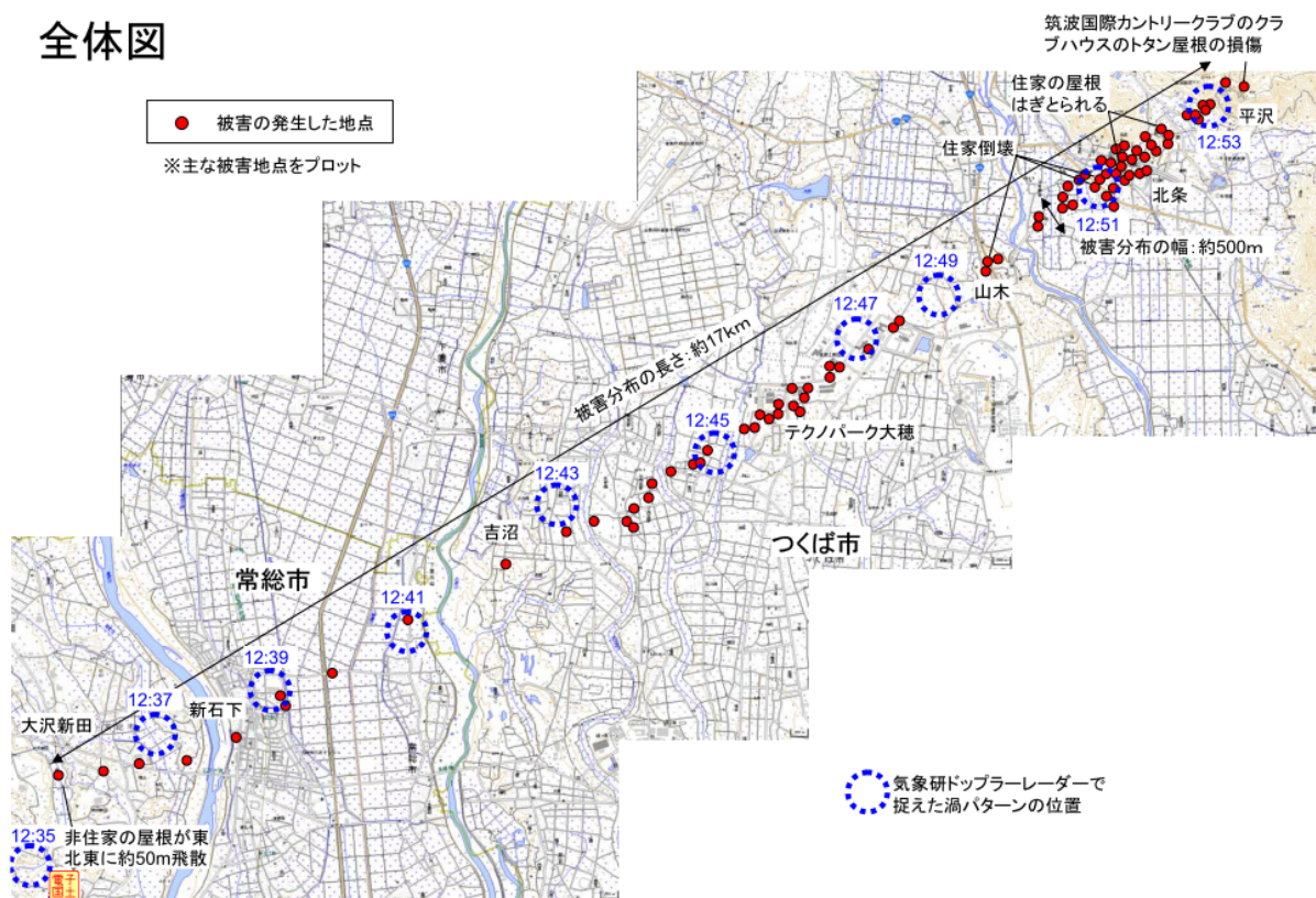
図1 気象研究所・水戸地方気象台・銚子地方気象台による現地調査で判明した突風被害の分布（赤プロット）、及び気象研究所ドップラーレーダーで捉えられた大気下層の渦の位置（青丸）。
