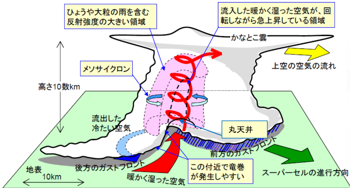
スーパーセルの模式図
