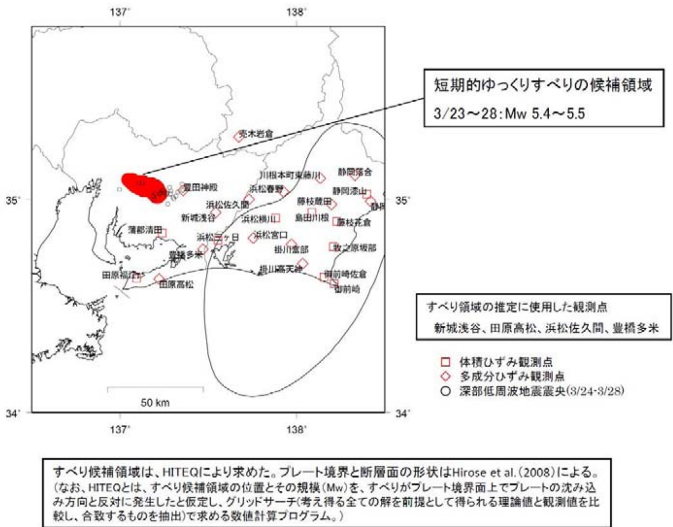
図6 3月23日から28日のひずみ変化から推定されるすべり領域
