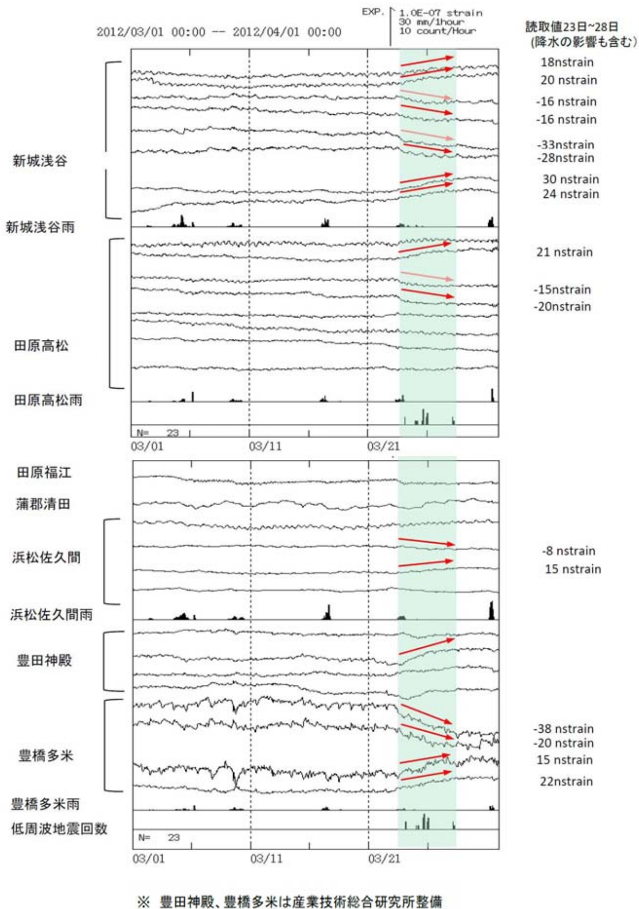
図5 愛知県における深部低周波地震活動(3月24日から28日まで)に伴うひずみ変化
