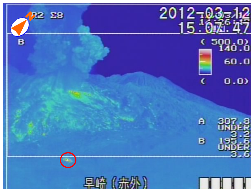
図 1 桜島 12 日 15 時 07 分の昭和火口の爆発的噴火の状況 （九州地方整備局大隅河川国道事務所の早崎カメラによる） 大きな噴石が 2 合目まで達しました。 赤丸が落下地点
