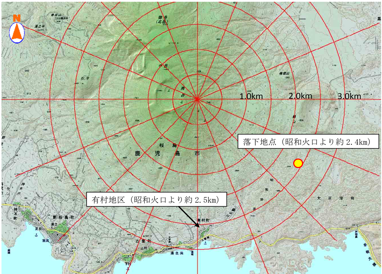
図2 桜島 12日15時07分の昭和火口の爆発的噴火による噴石落下地点 大きな噴石が2合目（昭和火口から2km付近）まで達しました。
