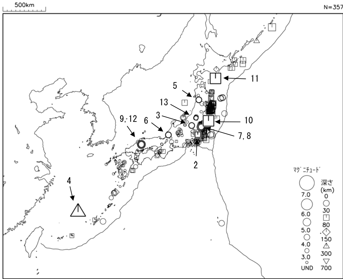
図 1 平成 23 年 11 月に震度 1 以上を観測した地震 (図中の番号は、3 ページの表の番号に対応する主な地震)
