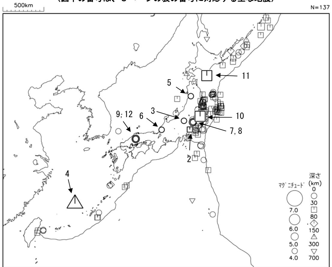
図 2 平成 23 年 11 月に発生した M4.0 以上の地震 (図中の番号は、3 ページの表の番号に対応する主な地震)
