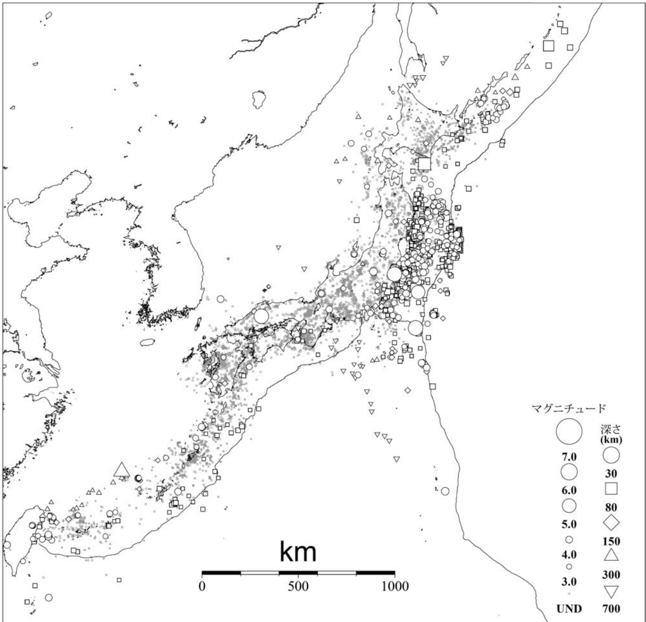
図3 気象庁が震源を決定した日本付近の平成23年11月の地震の震央分布 (M3.0以上の地震については白抜きで示す)
