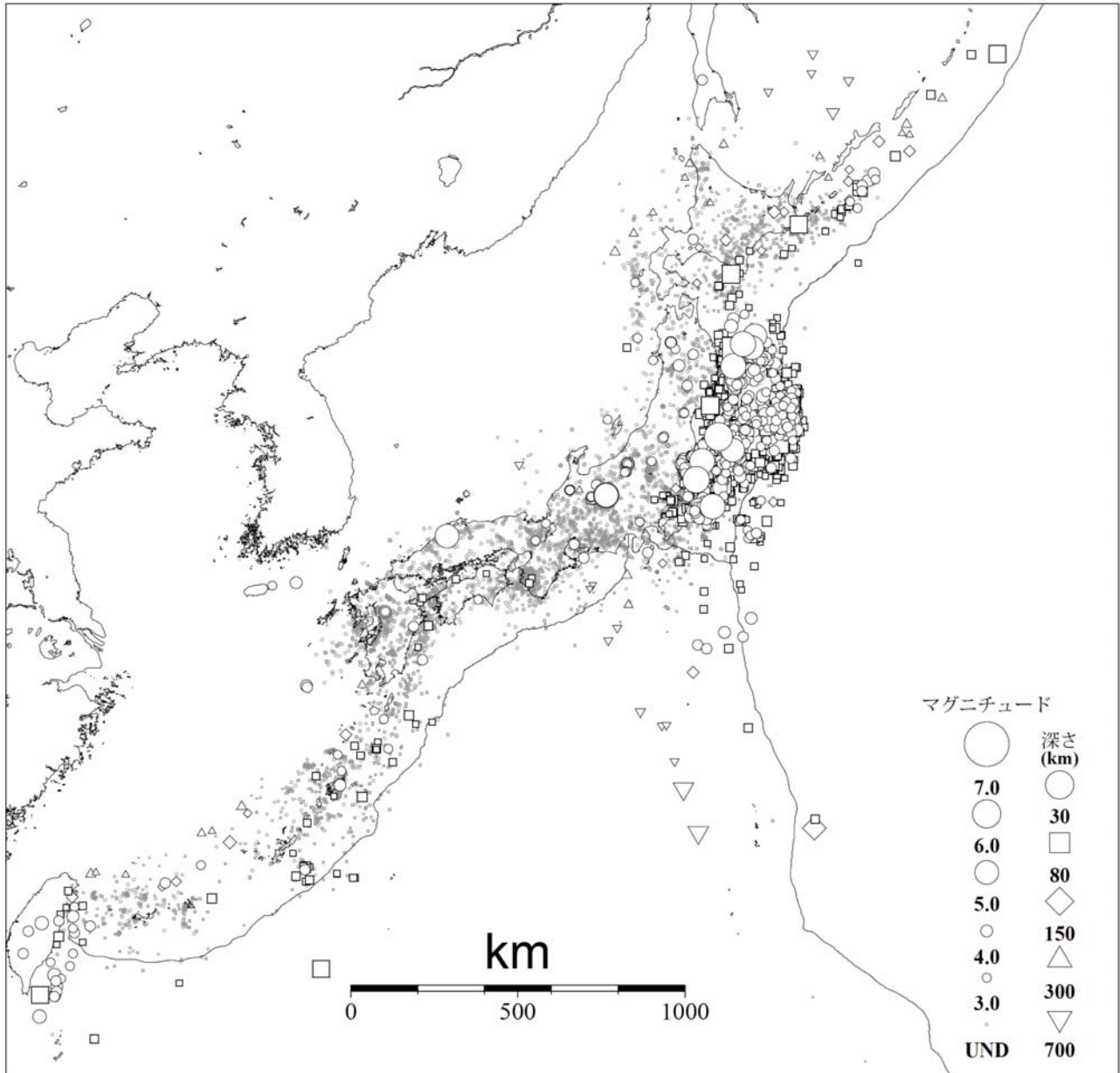
図3 気象庁が震源を決定した日本付近の平成23年6月の地震の震央分布 (M3.0以上の地震については白抜きで示す)
