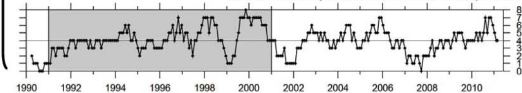
図3 東海地域の地震活動指数の推移 □：基準期間 ▲：地震活動指数（0-8）
