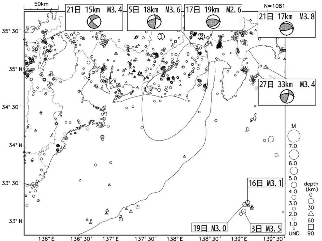
図1 震央分布図(2011年5月1日～31日:深さ0～90km、Mすべて。図中のナス型の領域は東海地震の想定震源域。)
