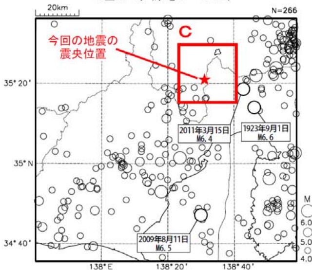
図6 5月17日に発生した山梨県中・西部の地震
