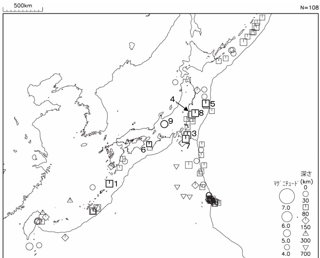
図2 平成23年2月に発生したM4.0以上の地震 (図中の番号は、2ページの表の番号に対応する地震)
