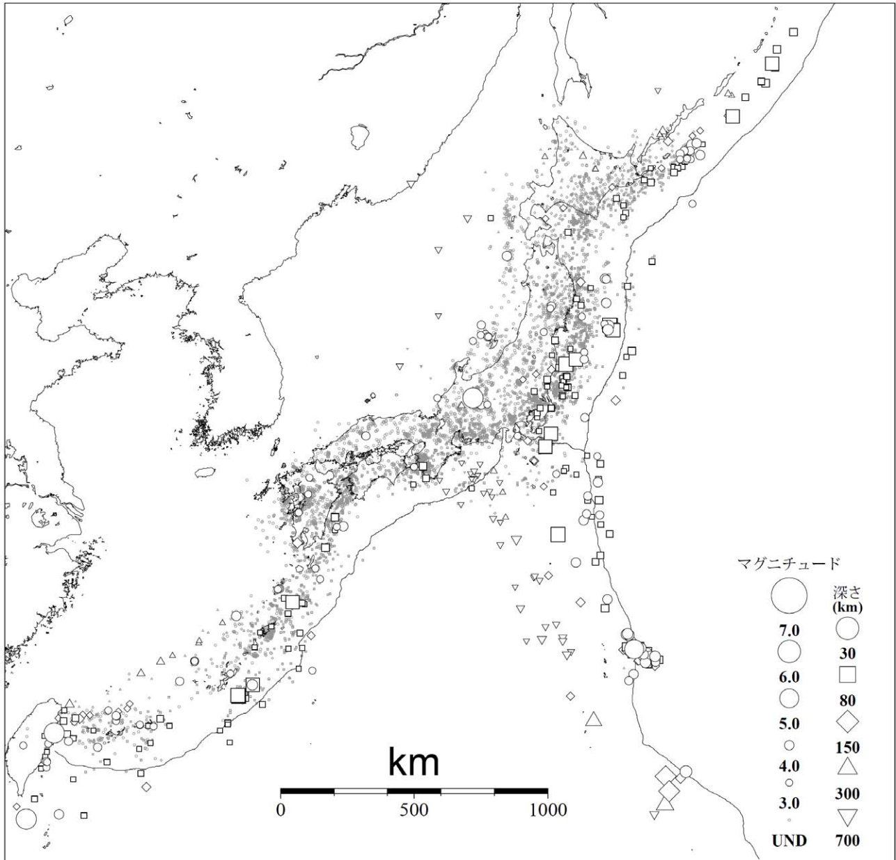
図3 気象庁が震源を決定した日本付近の平成23年2月の地震の震央分布 (M3.0以上の地震については白抜きで示す)
