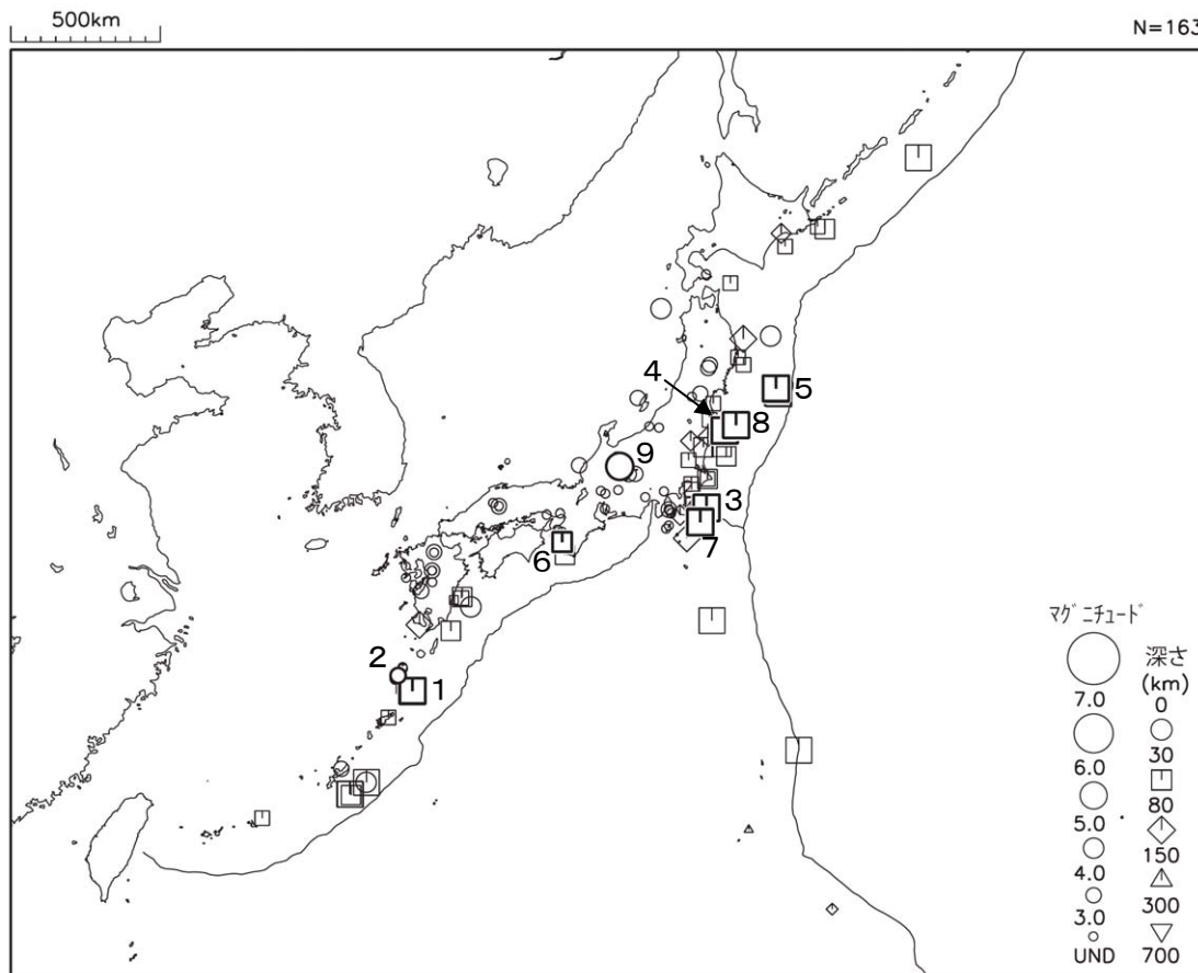
図1 平成23年2月に震度1以上を観測した地震 (図中の番号は、2ページの表の番号に対応する地震)
