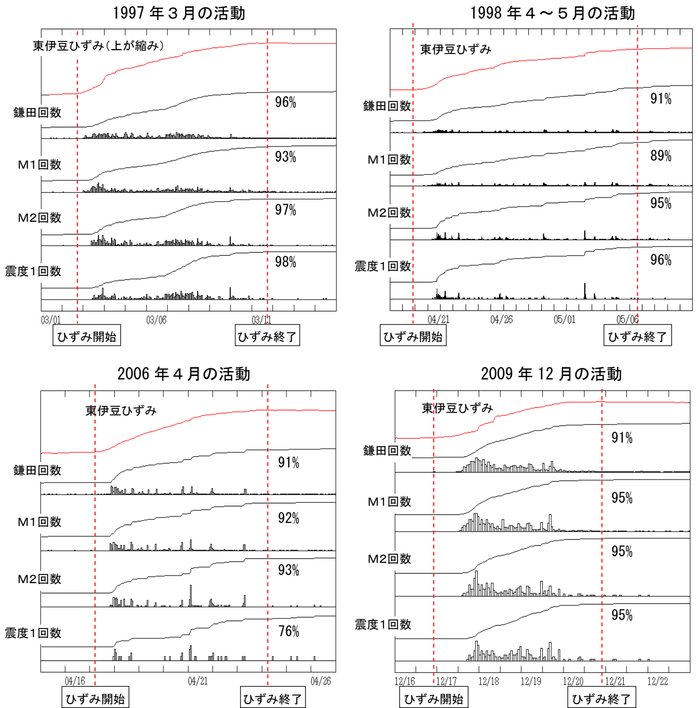
図20 ひずみ期間に発生した地震数（鎌田地震回数、M1回数、M2回数、震度1回数）の割合（鎌田の地震回数を基にした期間に発生した地震を100%とした）
