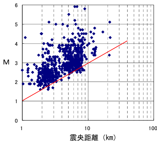
図18 伊東市大原における有感地震のMと震央距離（左）、伊東市大原からの震央距離（右）
