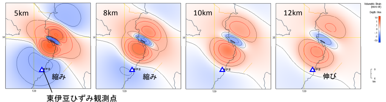
図8 マグマの深さによる、東伊豆のひずみ変化傾向の違い
