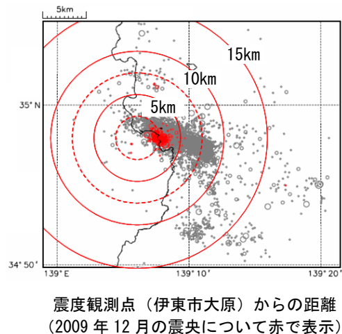
図18 伊東市大原における有感地震のMと震央距離（左）、伊東市大原からの震央距離（右）
