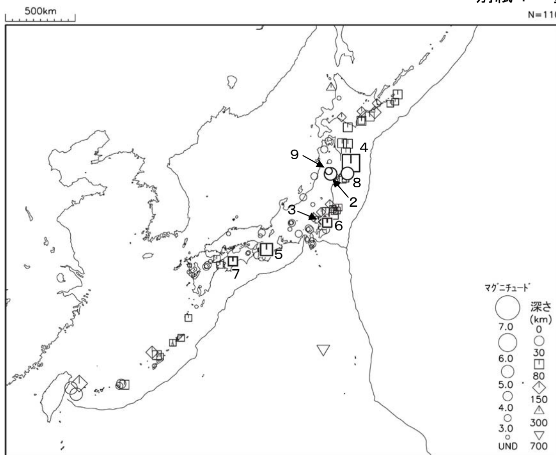
図1 平成22年7月に震度1以上を観測した地震 (図中の番号は、2ページの表の番号に対応する地震)
