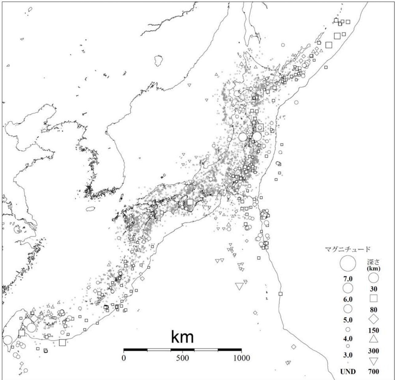
図3 気象庁が震源を決定した日本付近の平成22年7月の地震の震央分布 (M3.0以上の地震については白抜きで示す)
