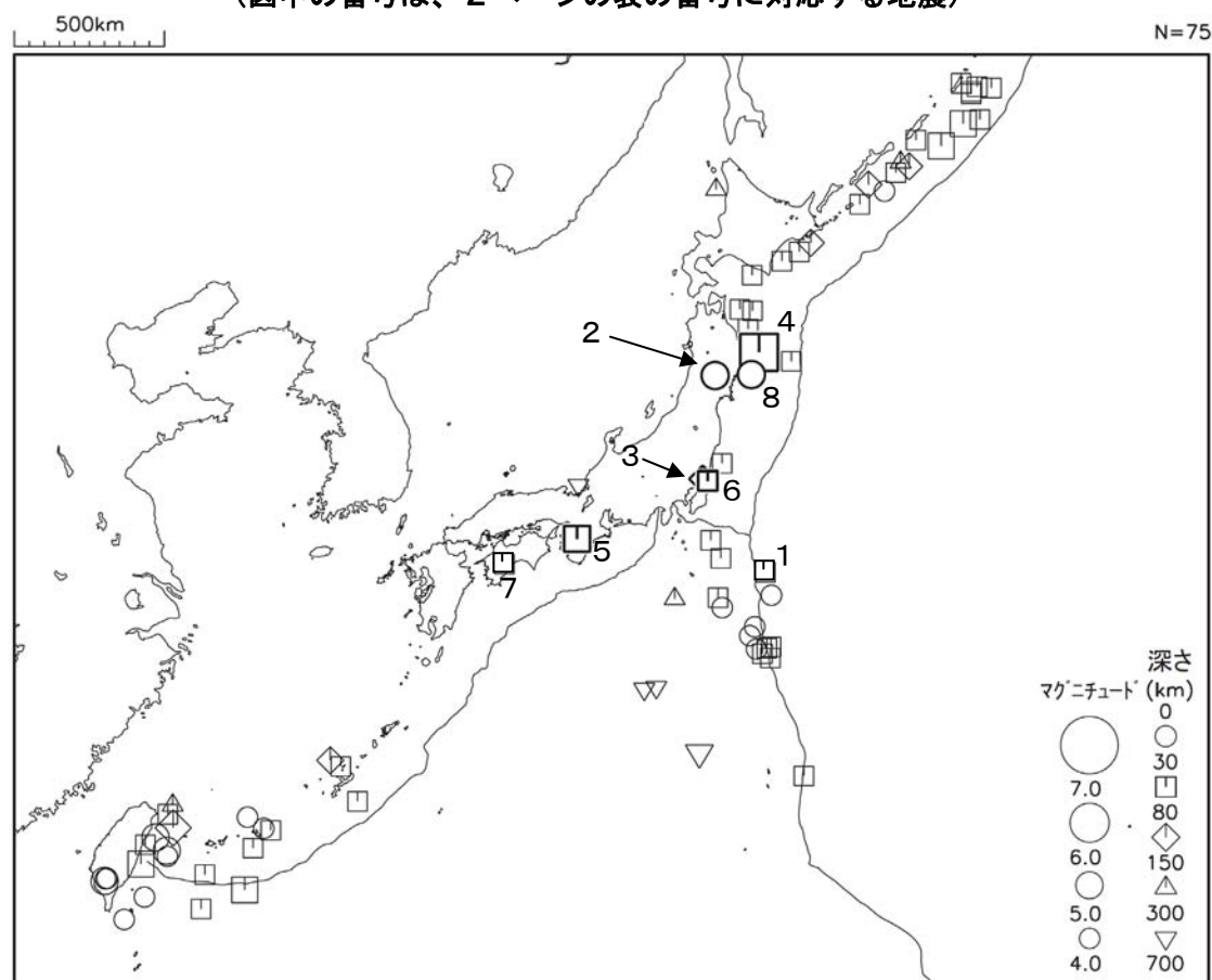
図2 平成22年7月に発生したM4.0以上の地震 (図中の番号は、2ページの表の番号に対応する地震)
