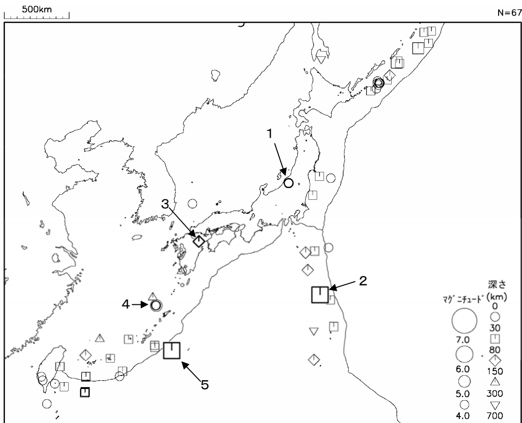
図2 平成22年5月に発生したM4.0以上の地震 (図中の番号は、2ページの表の番号に対応する地震)
