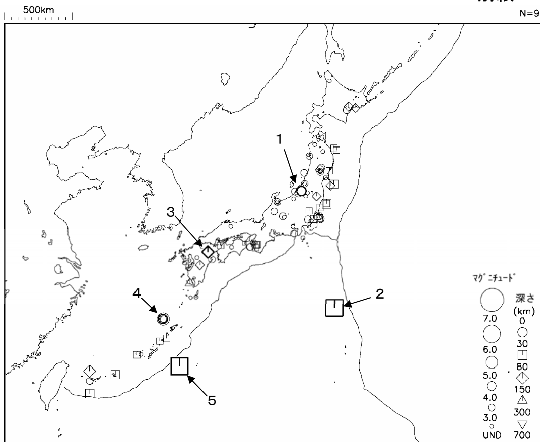
図1 平成22年5月に震度1以上を観測した地震 (図中の番号は、2ページの表の番号に対応する地震)
