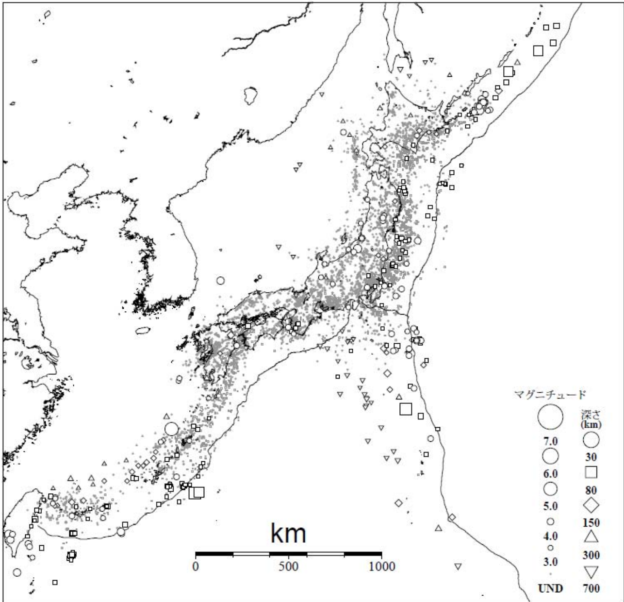
図3 気象庁が震源を決定した日本付近の平成22年5月の地震の震央分布 (M3.0以上の地震については白抜きで示す)
