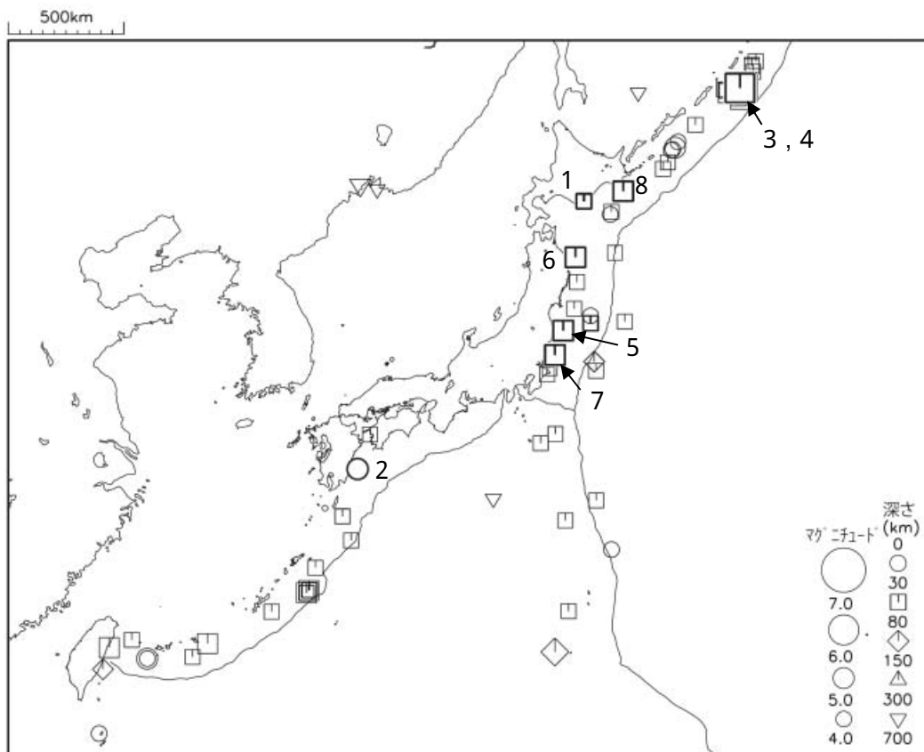
図2 平成 21 年 4 月に発生した M4.0 以上の地震 (図中の番号は、2 ページの表の番号に対応する地震)
