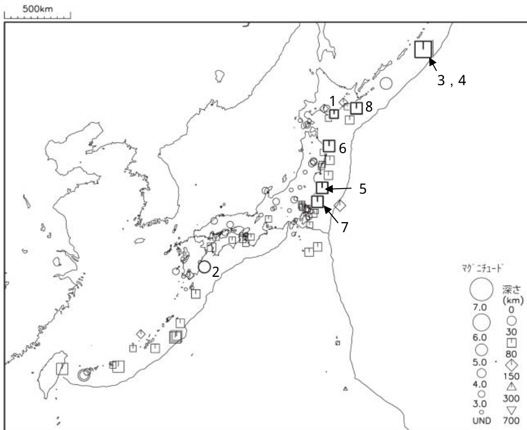
図1 平成 21 年 4 月に震度 1 以上を観測した地震 (図中の番号は、2 ページの表の番号に対応する地震)
