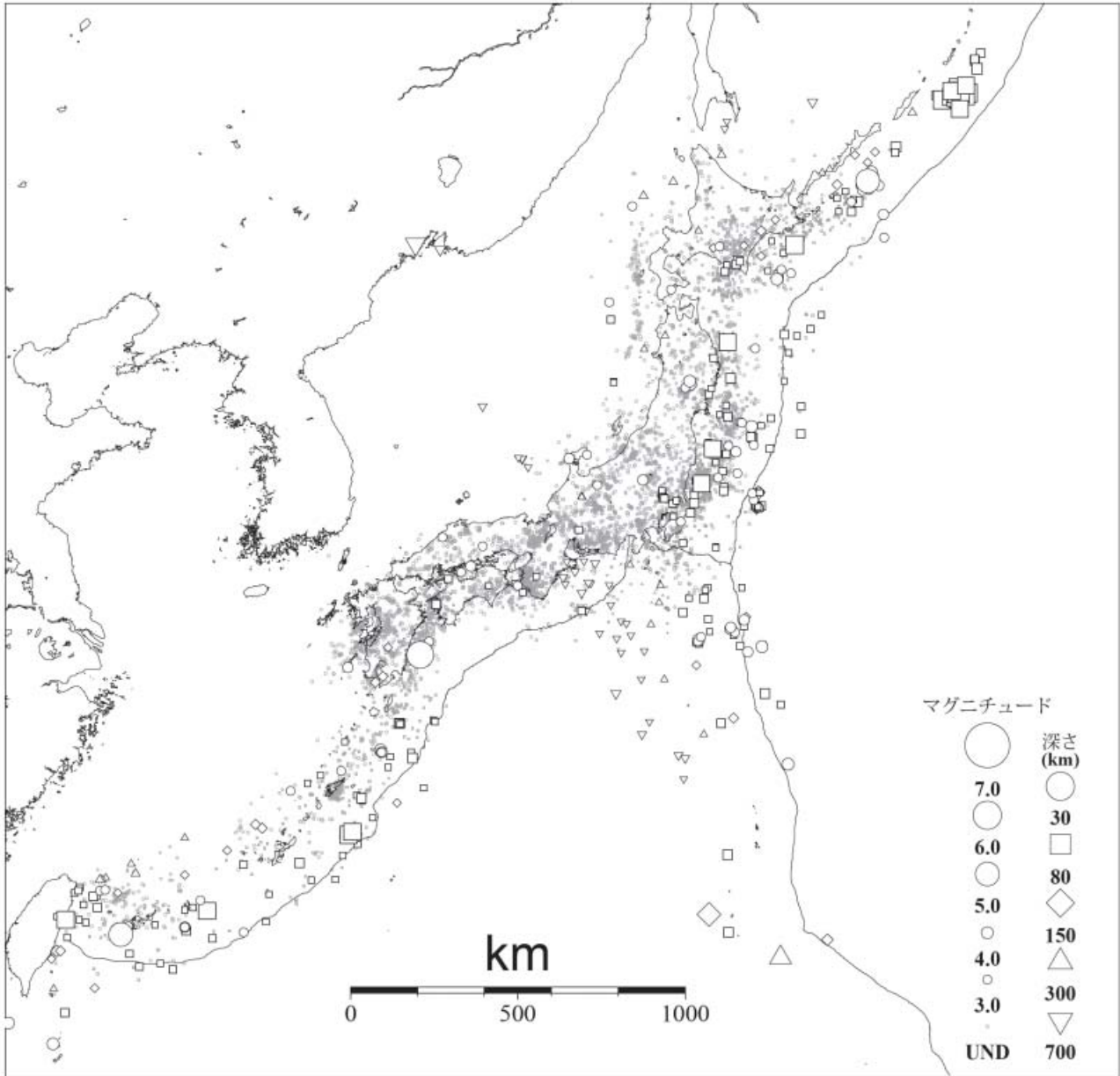
図3 気象庁が震源を決定した日本付近の平成 21 年 4 月の地震の震央分布 (M3.0 以上の地震については白抜きで示す)
