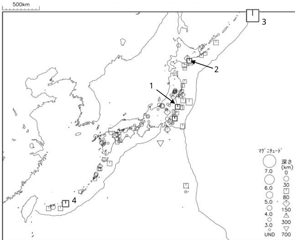
図1 平成 21 年 1 月に震度 1 以上を観測した地震 (図中の番号は、2 ページの表の番号に対応する地震)
