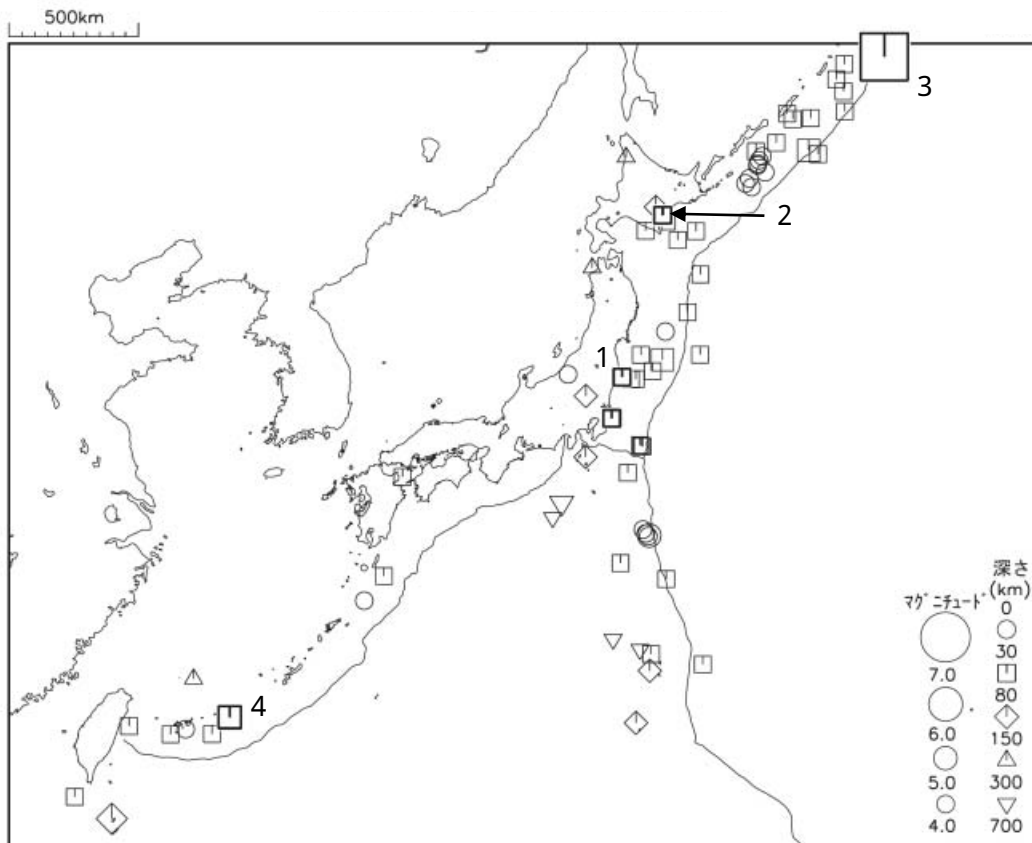
図2 平成 21 年 1 月に発生した M4.0 以上の地震 (図中の番号は、2 ページの表の番号に対応する地震)
