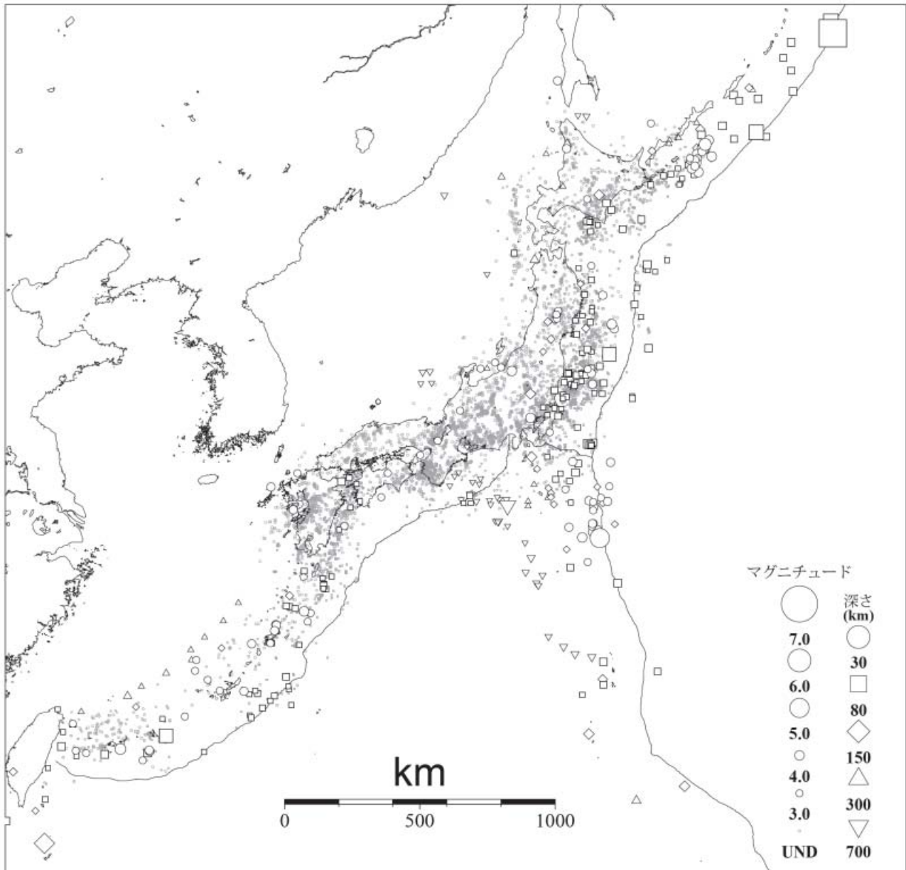
図3 気象庁が震源を決定した日本付近の平成 21 年 1 月の地震の震央分布 (M3.0 以上の地震については白抜きで示す)
