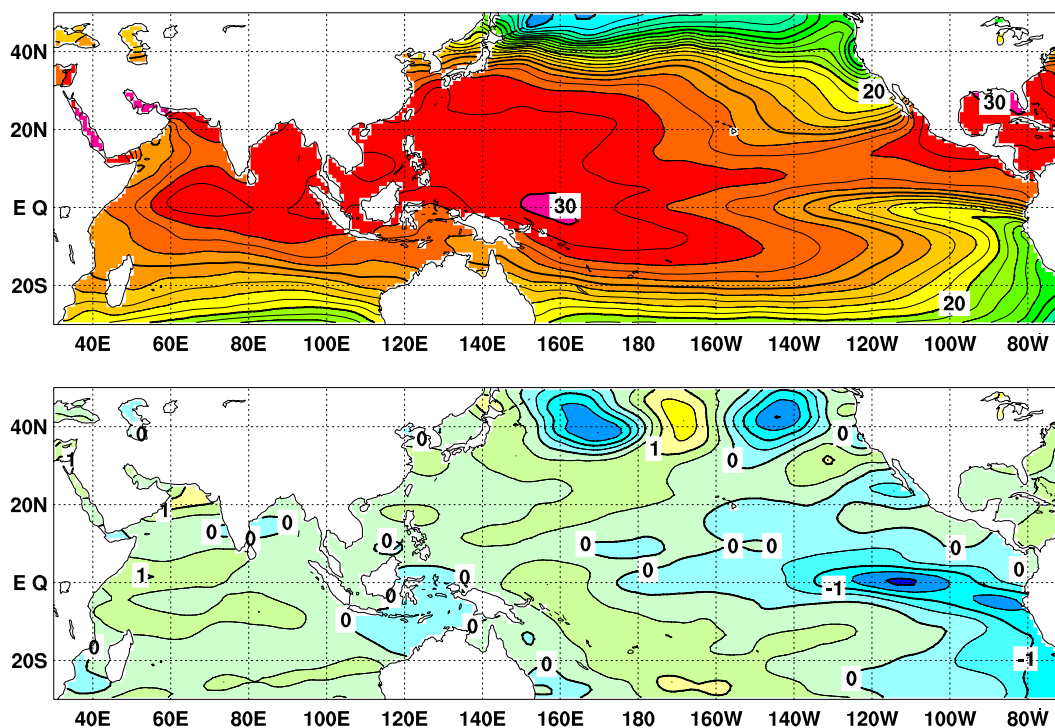
図 2 2007 年 8 月の海面水温図 ( 上 ) 及び平年偏差図 ( 下 )。海面水温図の太線は 5^{\circ}\text{C} 毎、細線は 1^{\circ}\text{C} 毎の、平年偏差図の太線は 1^{\circ}\text{C} 毎、細線は 0.5^{\circ}\text{C} 毎の等値線を示す ( 平年値は 1971 ~ 2000 年の 30 年平均値 )。
