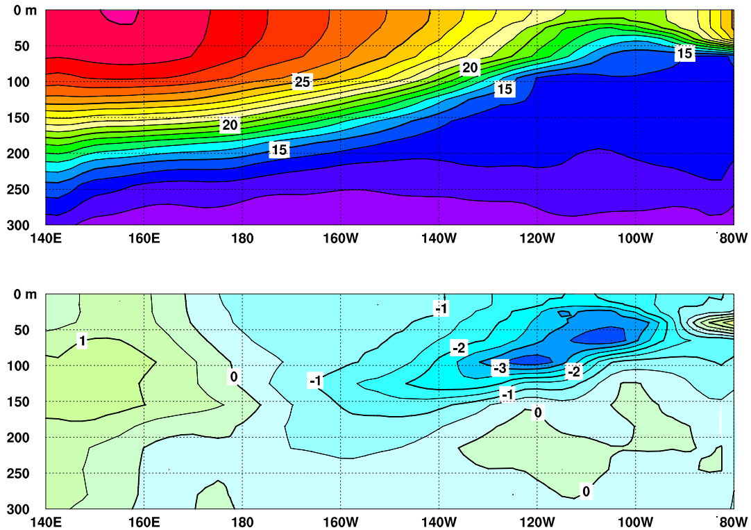
図3 2007年8月の太平洋の赤道に沿った水温(上)及び平年偏差(下)の断面図(海洋データ同化システムによる)。上図の等値線間隔は 1^{\circ}\text{C} 、下図の等値線間隔は 0.5^{\circ}\text{C} (平年値は1987~2006年の20年平均値)。
