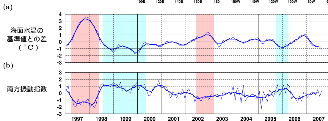
図1 エルニーニョ監視海域の海面水温の基準値との差( ^{\circ}\text{C} )(a)と南方振動指数(b)の推移(1997年1月~2007年8月)。折線は月平均値、滑らかな太線は5か月移動平均値を示す(海面水温の基準値はその年の前年までの30年間の各月の平均値、南方振動指数の年平均値は1971~2000年の30年平均値)。赤色の陰影はエルニーニョ現象の発生期間を、青色の陰影はラニーニャ現象の発生期間を示している。
