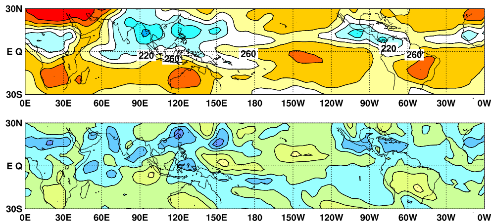
図 6 2007 年 8 月の外向き長波放射量 (OLR) ( 上 ) 及び年偏差 ( 下 ) の分布図。OLR の値が小さいほど、対流活動が活発であることを示す。上図は 20\text{W}/\text{m}^2 毎、下図は 10\text{W}/\text{m}^2 毎に等値線を描いている ( 年偏差は 1979 ~ 2004 年の 26 年平均値 )。OLR データは米国海洋大気庁 ( NOAA ) から提供されたものである。
